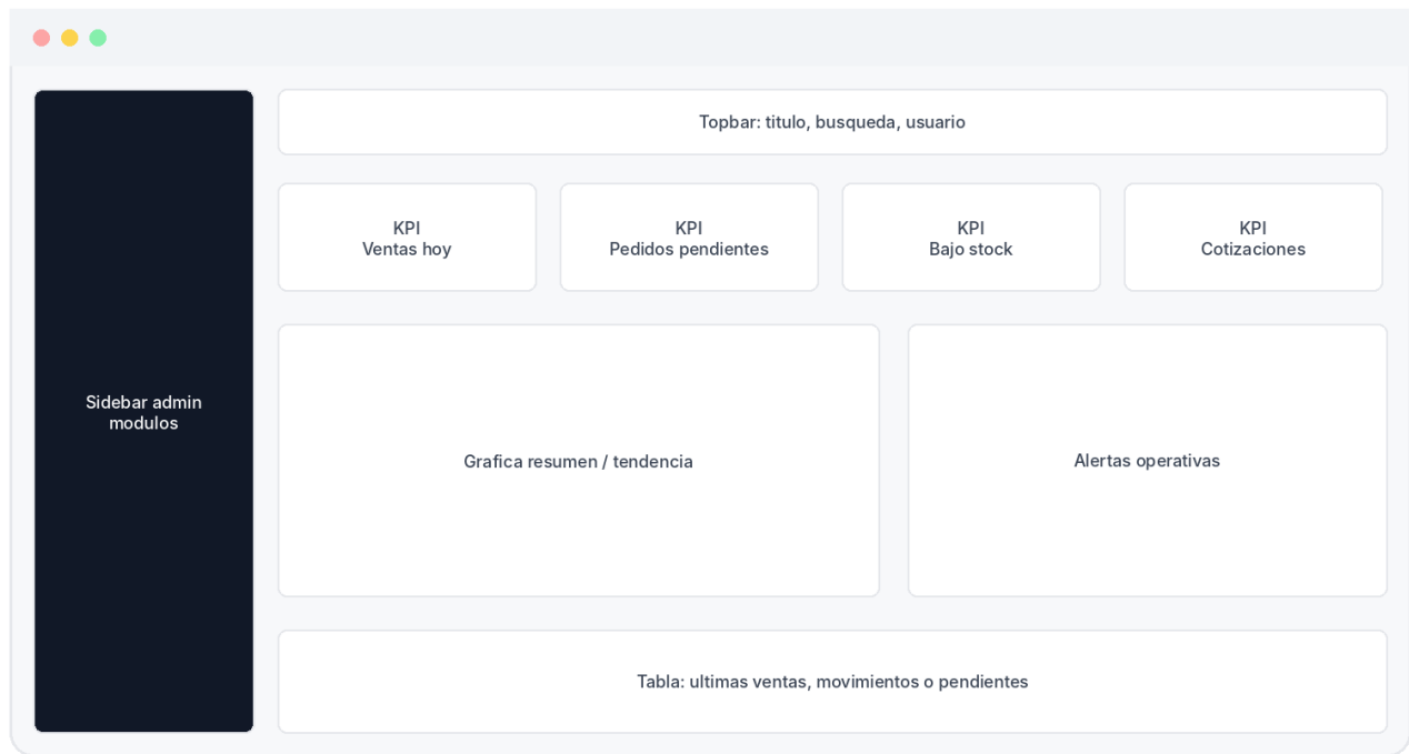
Figura 8. Wireframe técnico - Dashboard administrativo.
