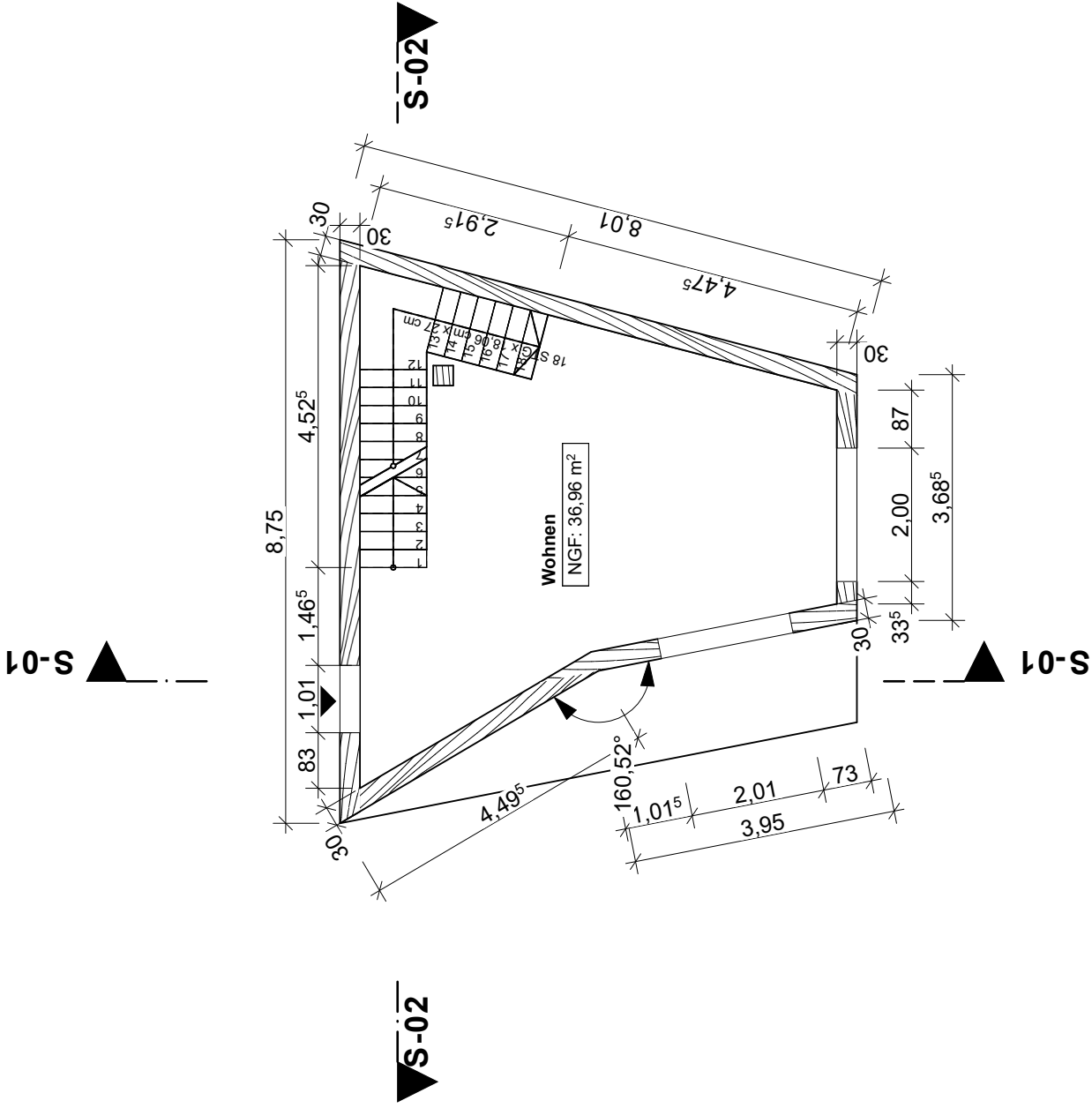
Grundriss 1.OG
