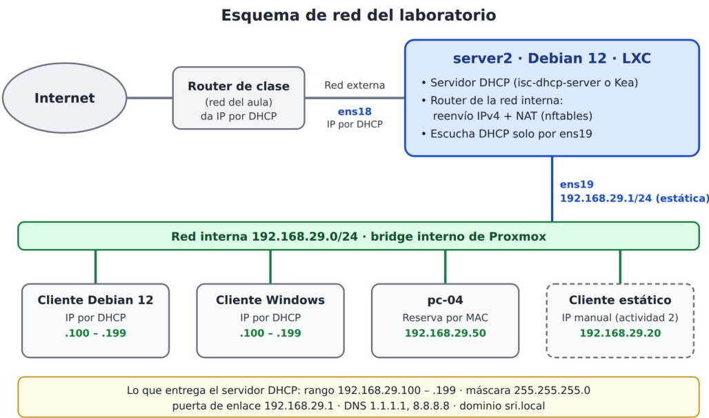
Esquema de red del laboratorio
