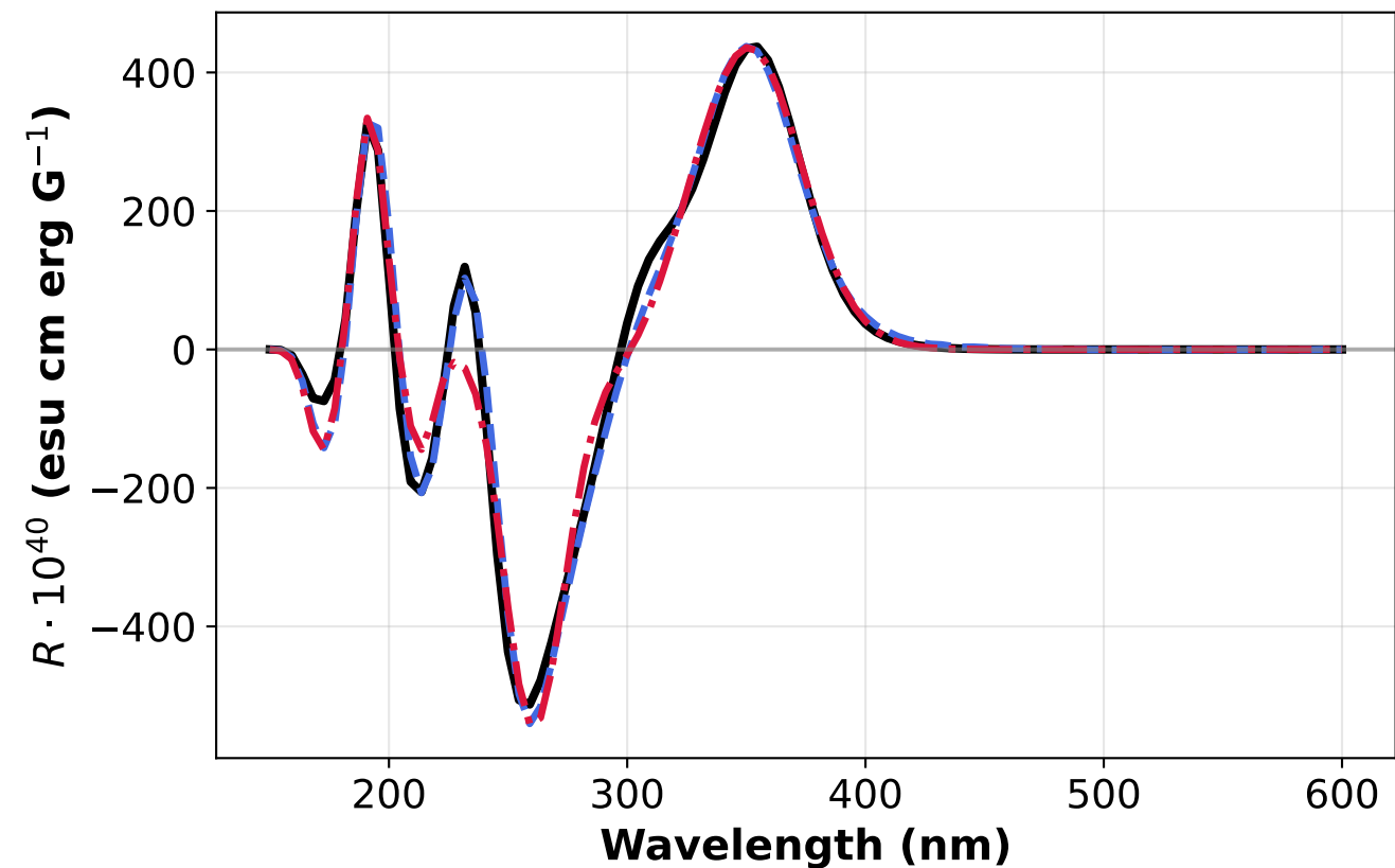
6Heliceno_6-CN MAE (E2E/PINN): 14.3 / 18.5 | Cos: 0.992 / 0.984
