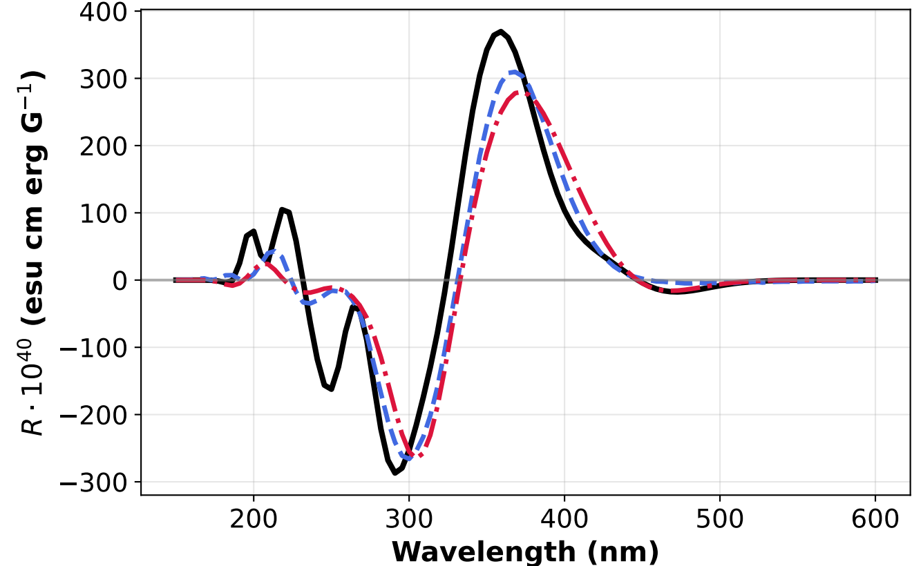
6Heliceno_1-CHO_5-CHO_4-CHO_9-NO2 MAE (E2E/PINN): 30.7 / 40.6 | Cos: 0.933 / 0.879
