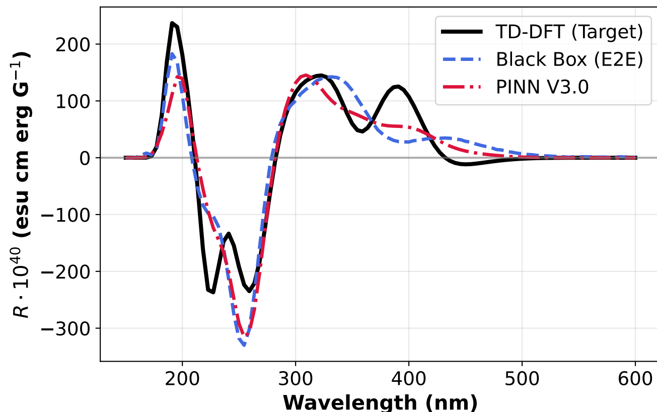
6Heliceno_6-SH_14-OMe_2-OMe_9-NH2 MAE (E2E/PINN): 25.8 / 29.0 | Cos: 0.978 / 0.966
