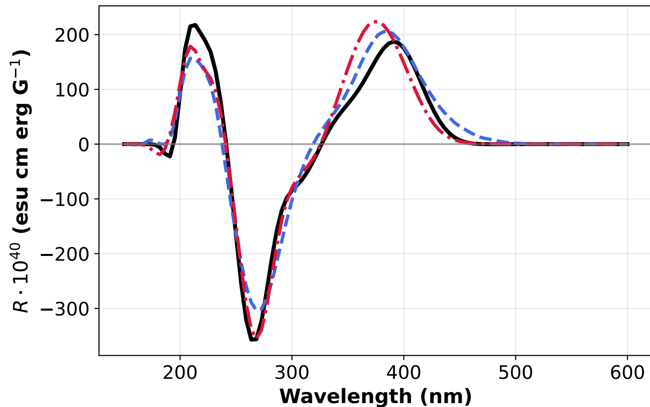
6Heliceno_1-cloro_2-fluor_3-bromo_4-bromo_5-yodo_6-fluor MAE (E2E/PINN): 19.7 / 17.7 | Cos: 0.971 / 0.971
