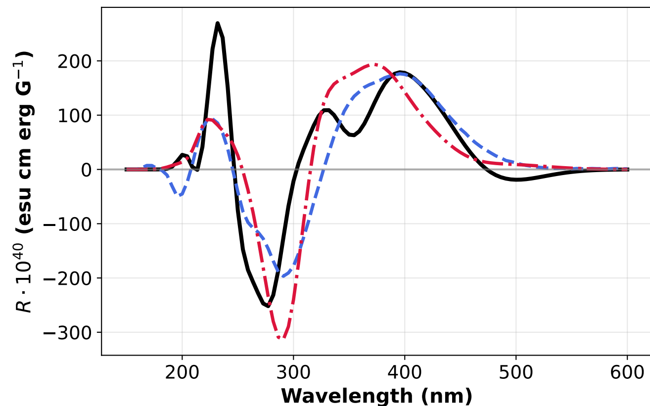
6Heliceno_2-OH_8-NH2_14-OH MAE (E2E/PINN): 22.2 / 18.7 | Cos: 0.986 / 0.988
