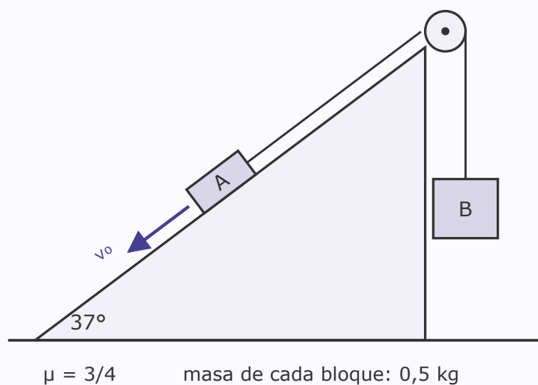
Figura 3: Bloque A sobre un plano inclinado 37^\circ , unido por una cuerda que pasa por una polea al bloque B, que cuelga.
