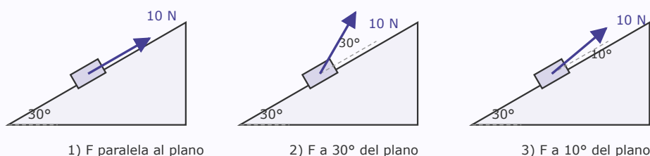
Figura 1: Las tres experiencias del problema 2: la fuerza de 10 N se aplica paralela al plano, formando 30^\circ con él y formando 10^\circ con él.
