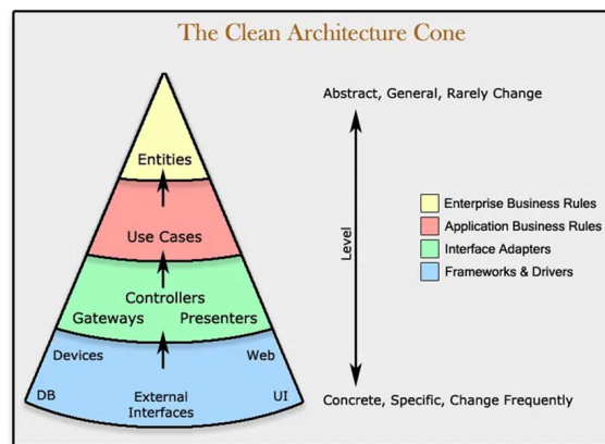
Figura 3.5: Esquema Clean Architecture en forma de Cono Adaptado de Martin (2012)
