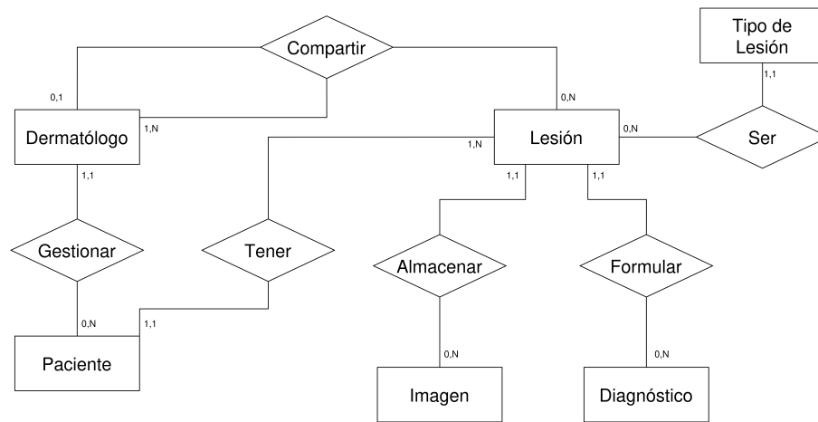
Figura 3.6: Modelo de Entidad Relacional MER
