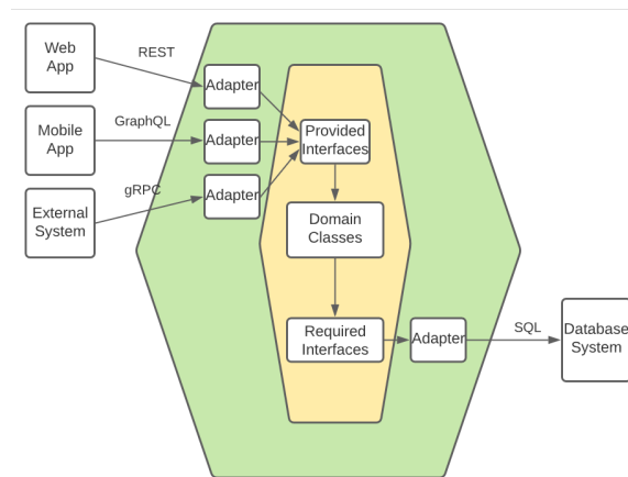
Figura 3.3: Esquema de la Arquitectura Hexagonal (Puertos y Adaptadores). Se observa el dominio en el centro, los puertos en los lados del hexágono y los adaptadores conectados a ellos. Imagen adaptada de CockburnCockburn 2005.
