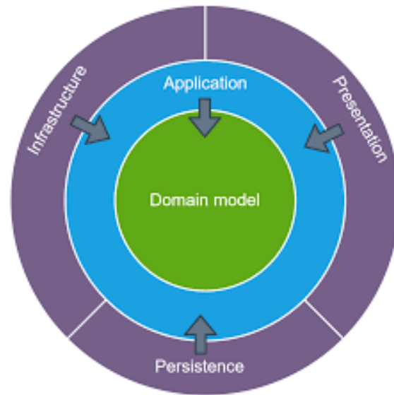
Figura 3.4: Esquema Onion Architecture, Tomado de Palermo (2008)
