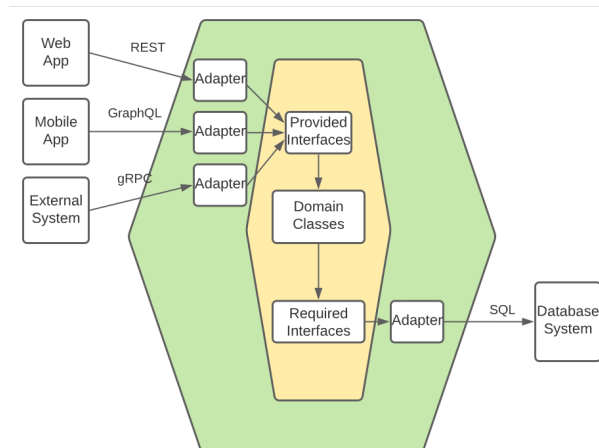
Figura 3.3: Esquema de la Arquitectura Hexagonal (Puertos y Adaptadores). Se observa el dominio en el centro, los puertos en los lados del hexágono y los adaptadores conectados a ellos. Imagen adaptada de Cockburn [6].
