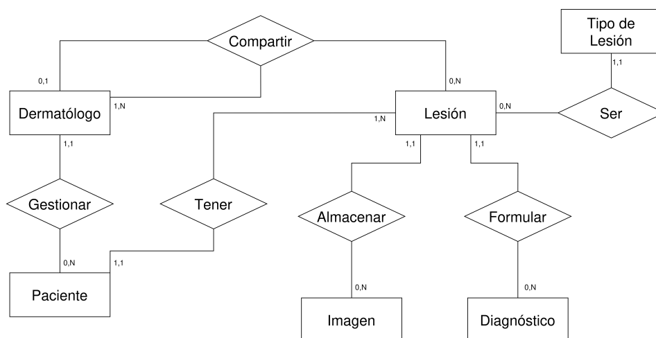
Figura 3.6: Modelo de Entidad Relacional MER
