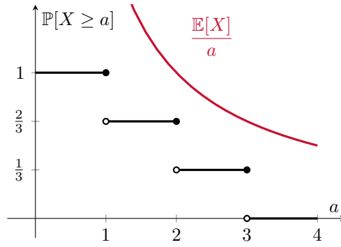
Figura 2.1: Desigualdad de Markov's en el Ejemplo 2.4.
