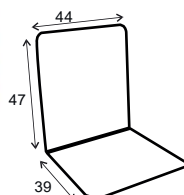
ESPESOR 20MM
