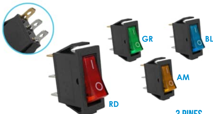
3 PINES 12V-20A
