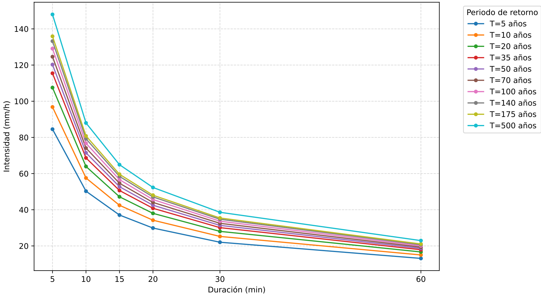
Curvas IDF — YANTAC (CO) Método de Dick y Peschke
