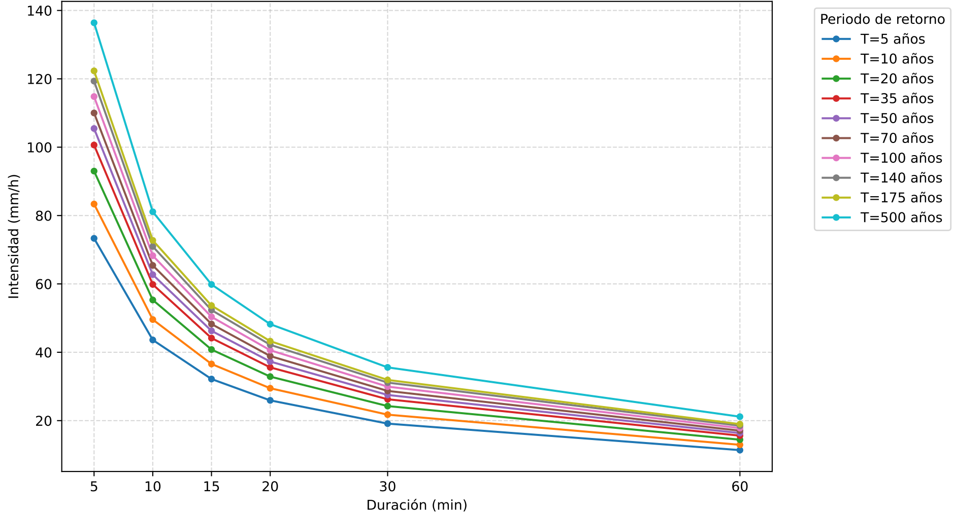
Curvas IDF — PIRCA (CO) Método de Dick y Peschke
