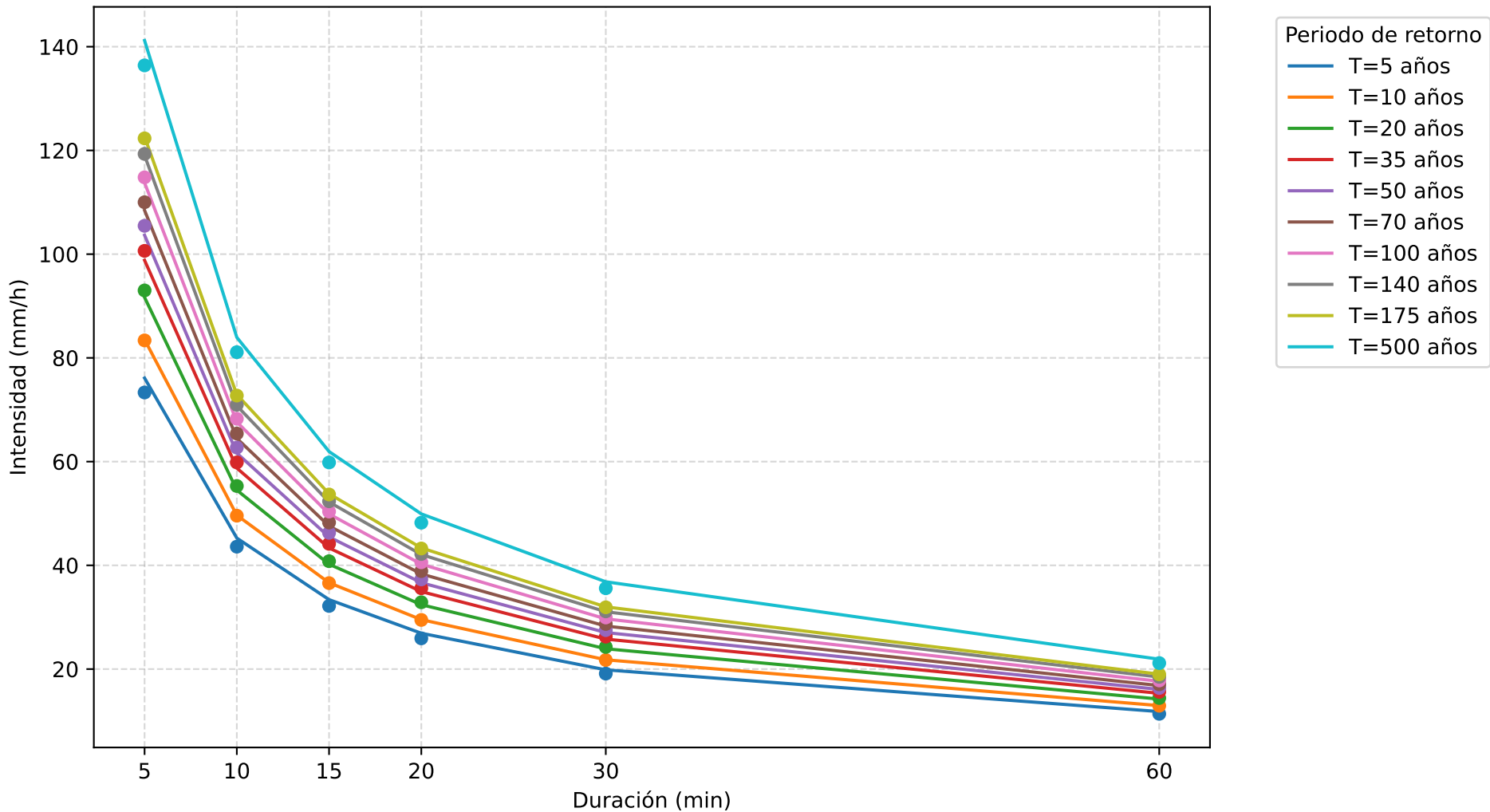
Curvas IDF ajustadas — PIRCA (CO) I = 205.055 \cdot Tr^{0.134185} / t^{0.750001}
