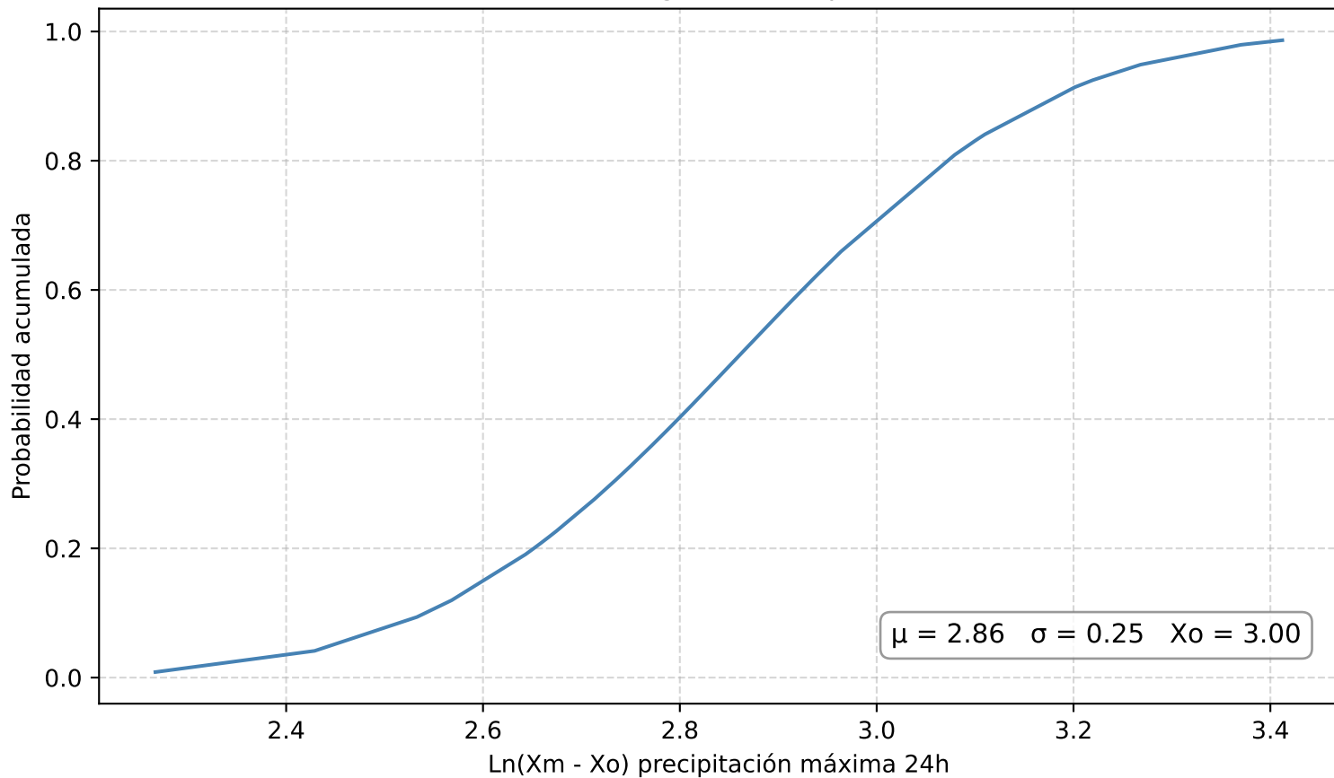
Distribución Log-Normal 3 parámetros
