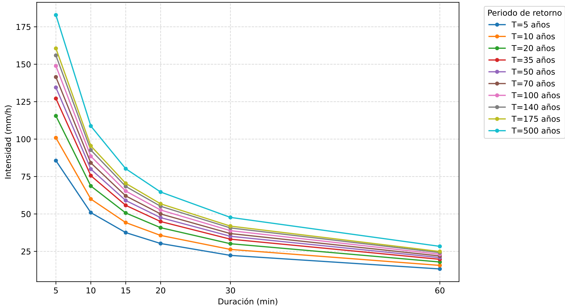
Curvas IDF — CANTA (CO) Método de Dick y Peschke
