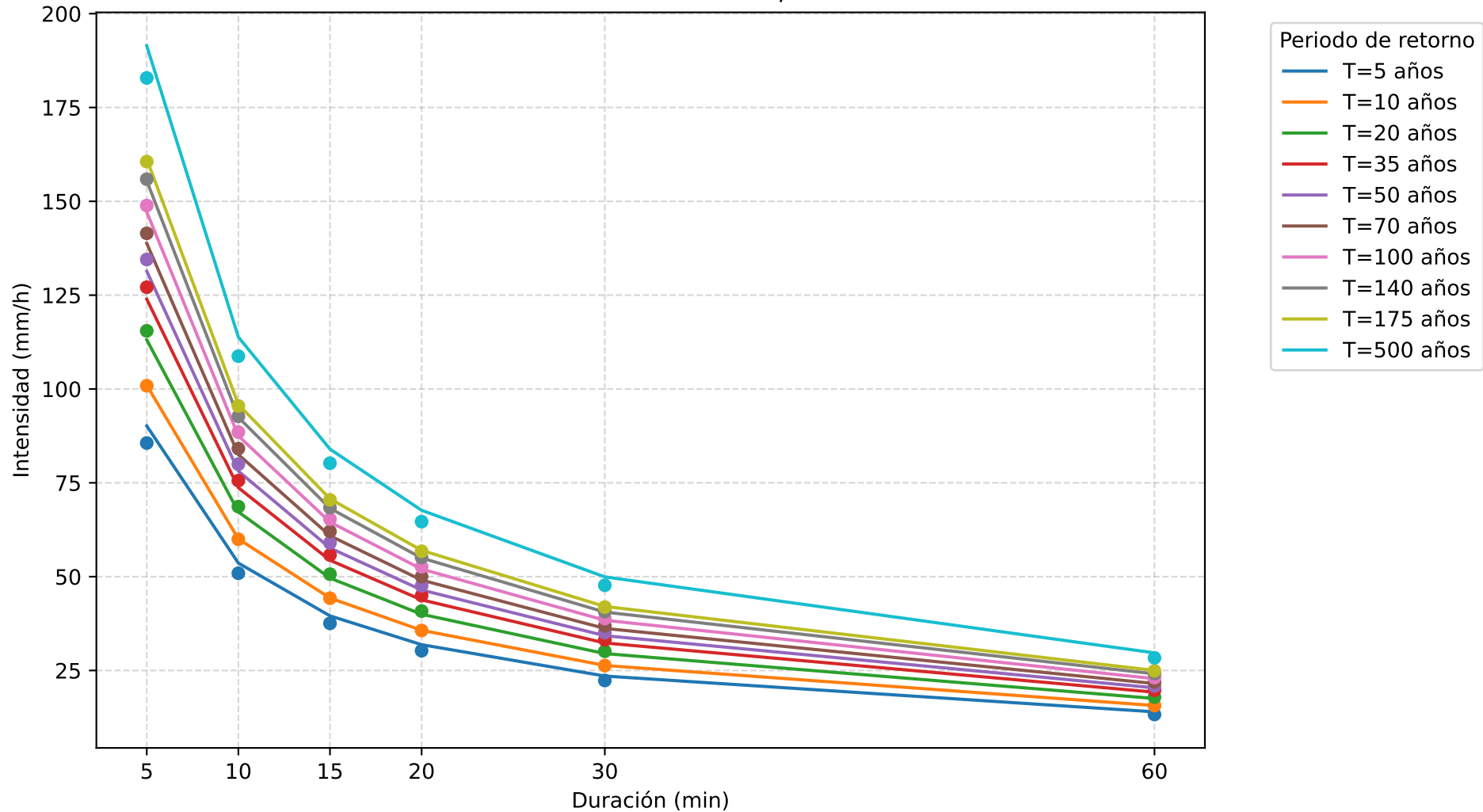
Curvas IDF ajustadas — CANTA (CO) I = 231.7408 \cdot Tr^{0.163485} / t^{0.75}
