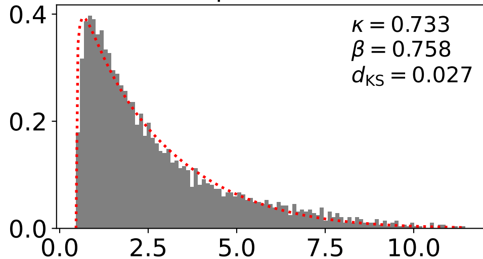
Epoch = 140
