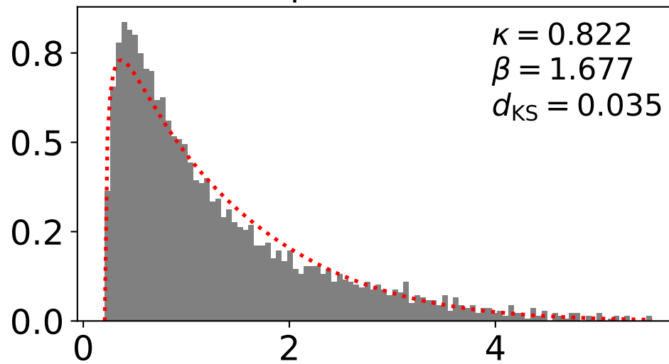
Epoch = 160
