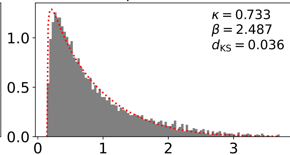
Epoch = 180
