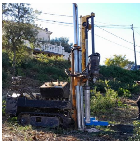
Fotografia 2. Vista de la màquina utilitzada per a la realització del sondeig a rotació.
