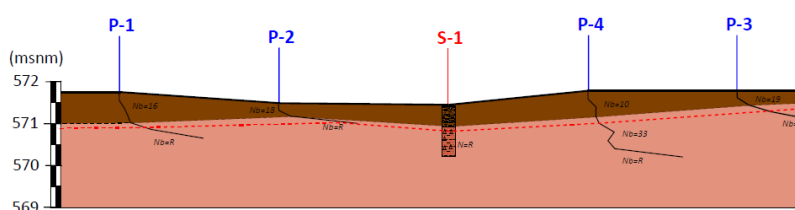
Figura 5. Tall de correlació.
