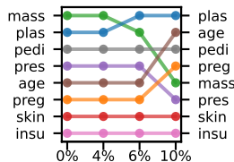
(P) DALEX | DT ( \sum C : 2.38)
