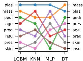
(D) EXIRT | Model Dependence ARD: 5.05
