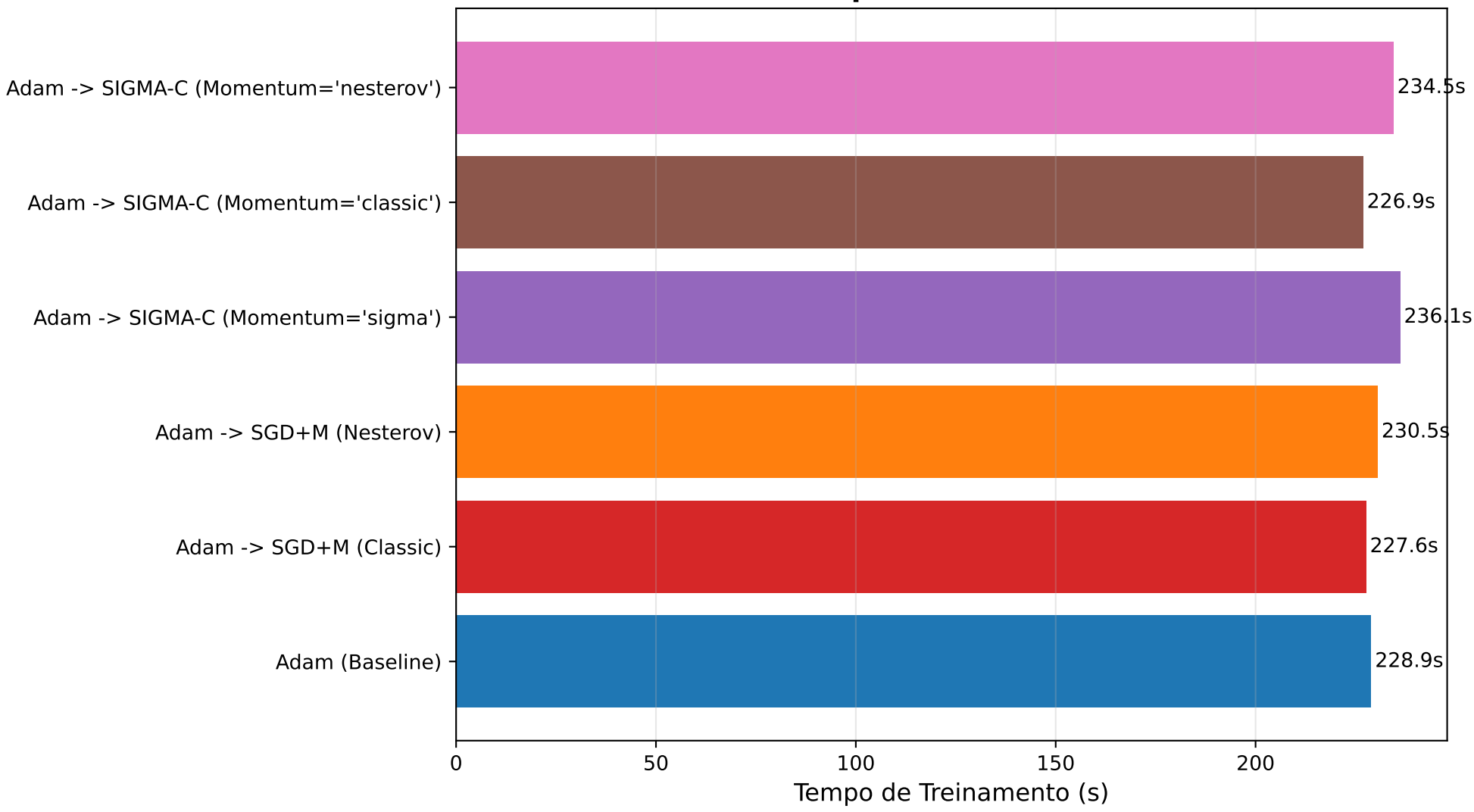
Eficiência Computacional (Redes Neurais)
