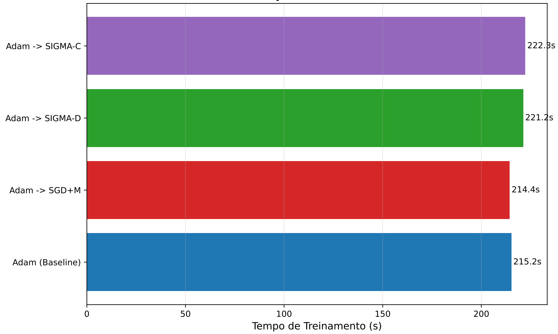
Eficiência Computacional (Redes Neurais)
