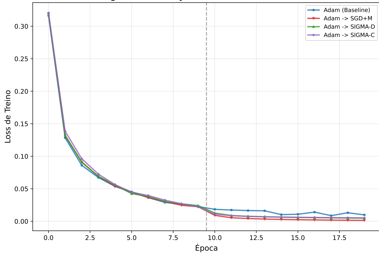
Convergência no Conjunto de Treino (Redes Neurais)
