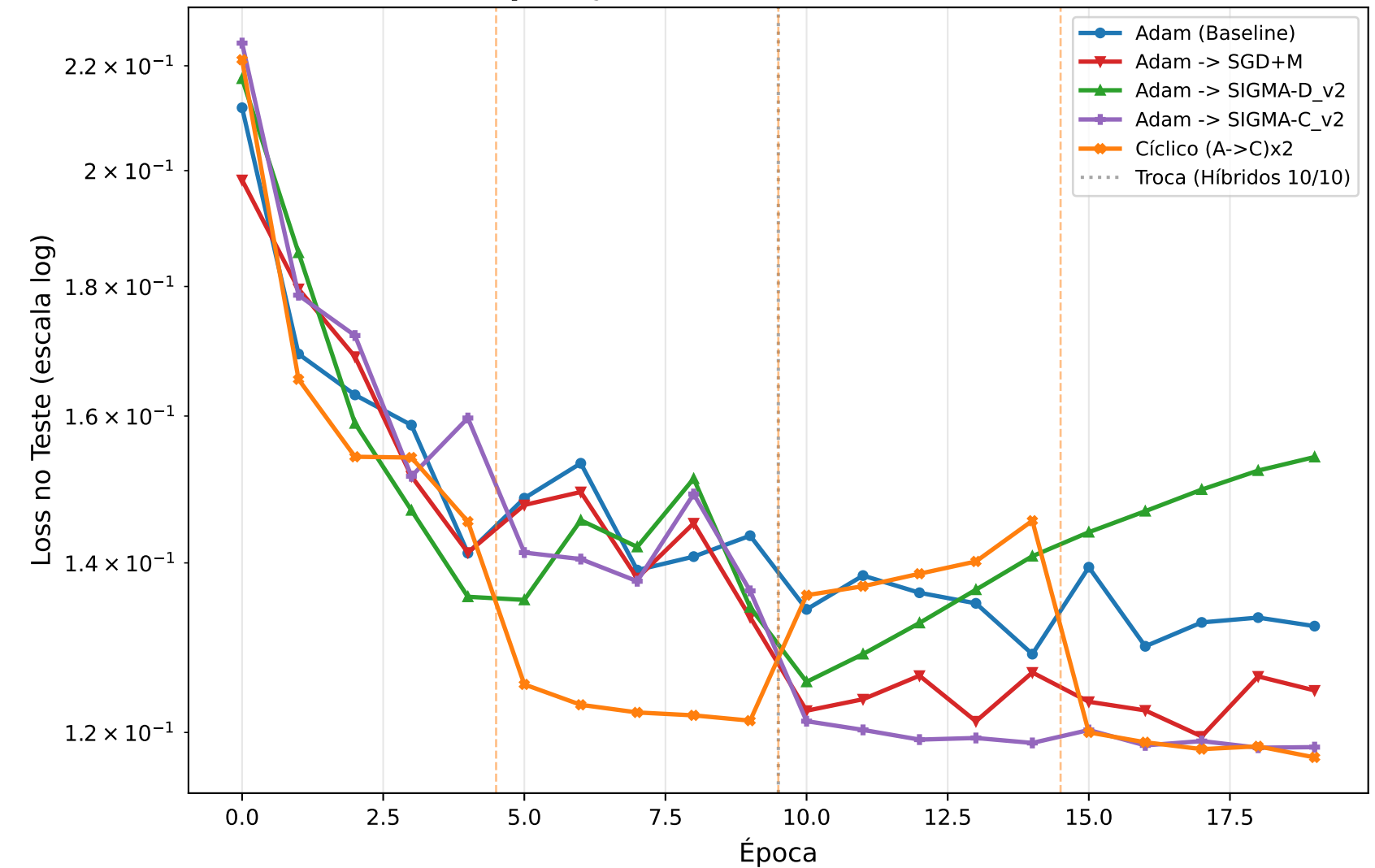
Eficiência Computacional v2 (Redes Neurais)
