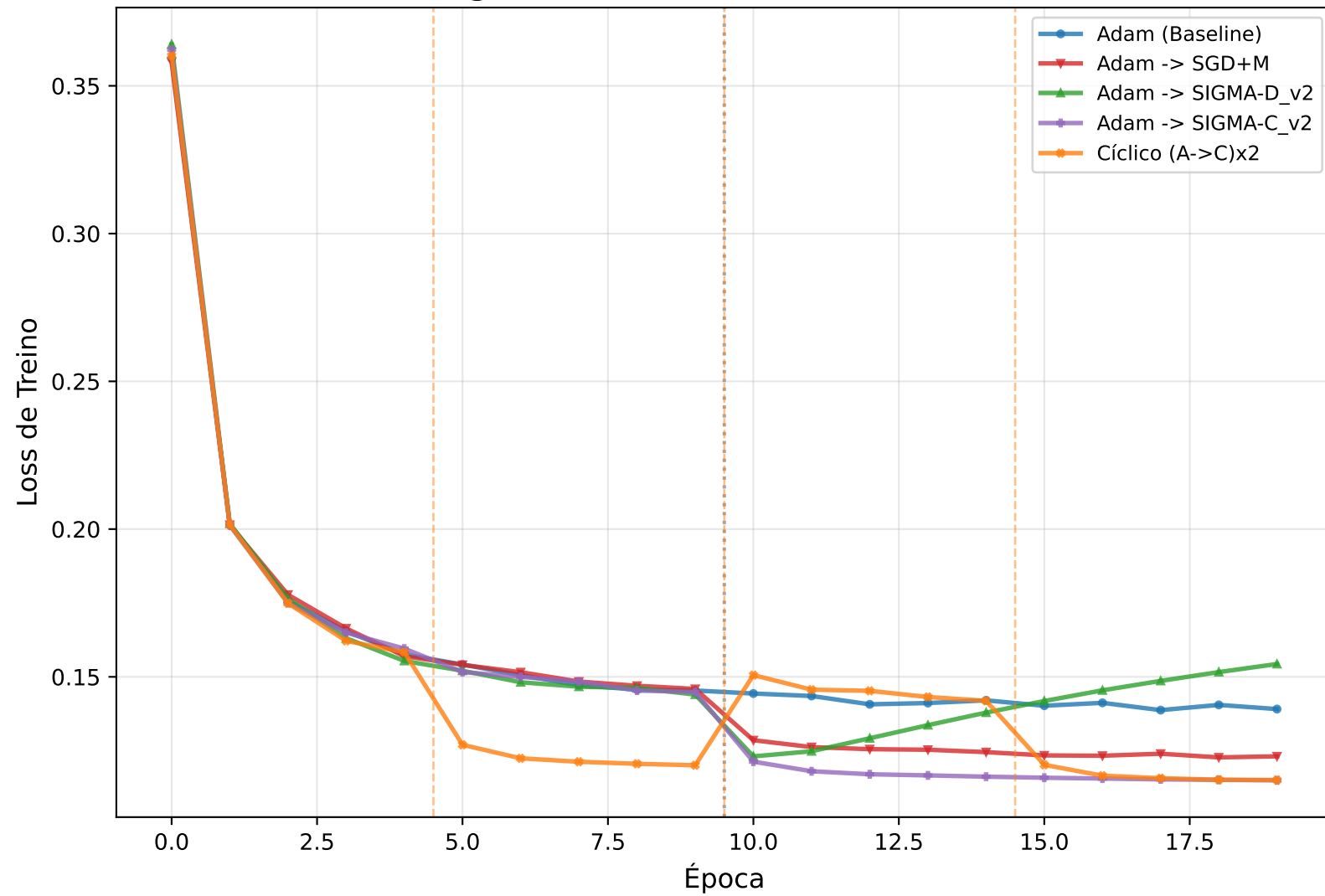
Convergência no Treino v2 (Redes Neurais)
