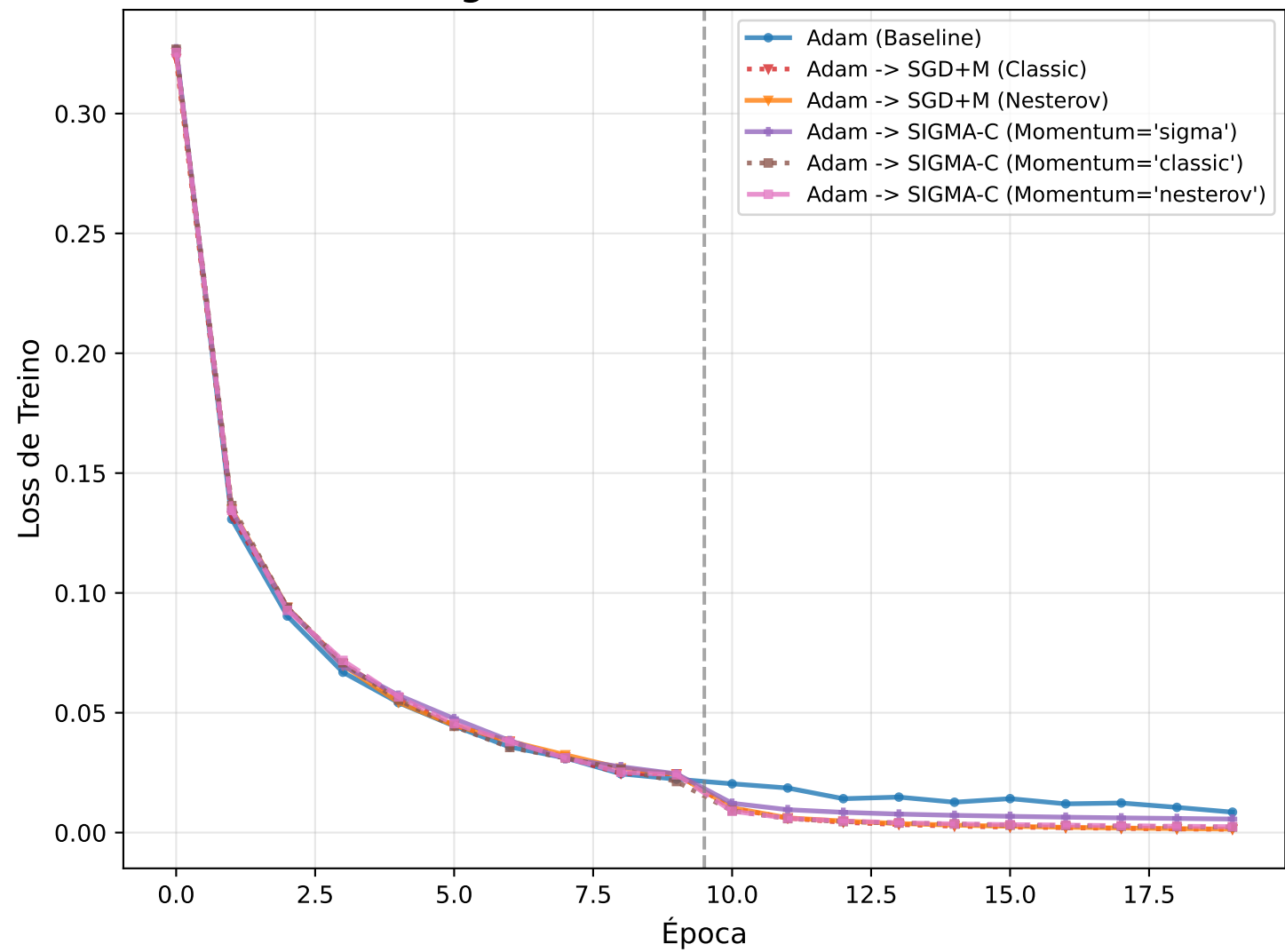
Convergência no Treino (Redes Neurais)
