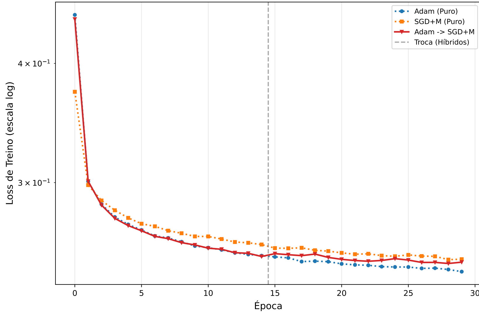
Regressão Logística v2.1: Convergência
