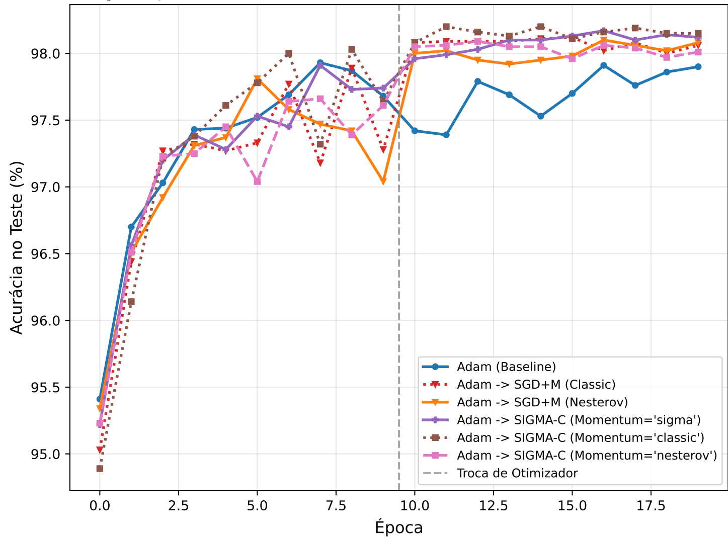
Comparação de Acurácia: Modos de Momentum (Redes Neurais)
