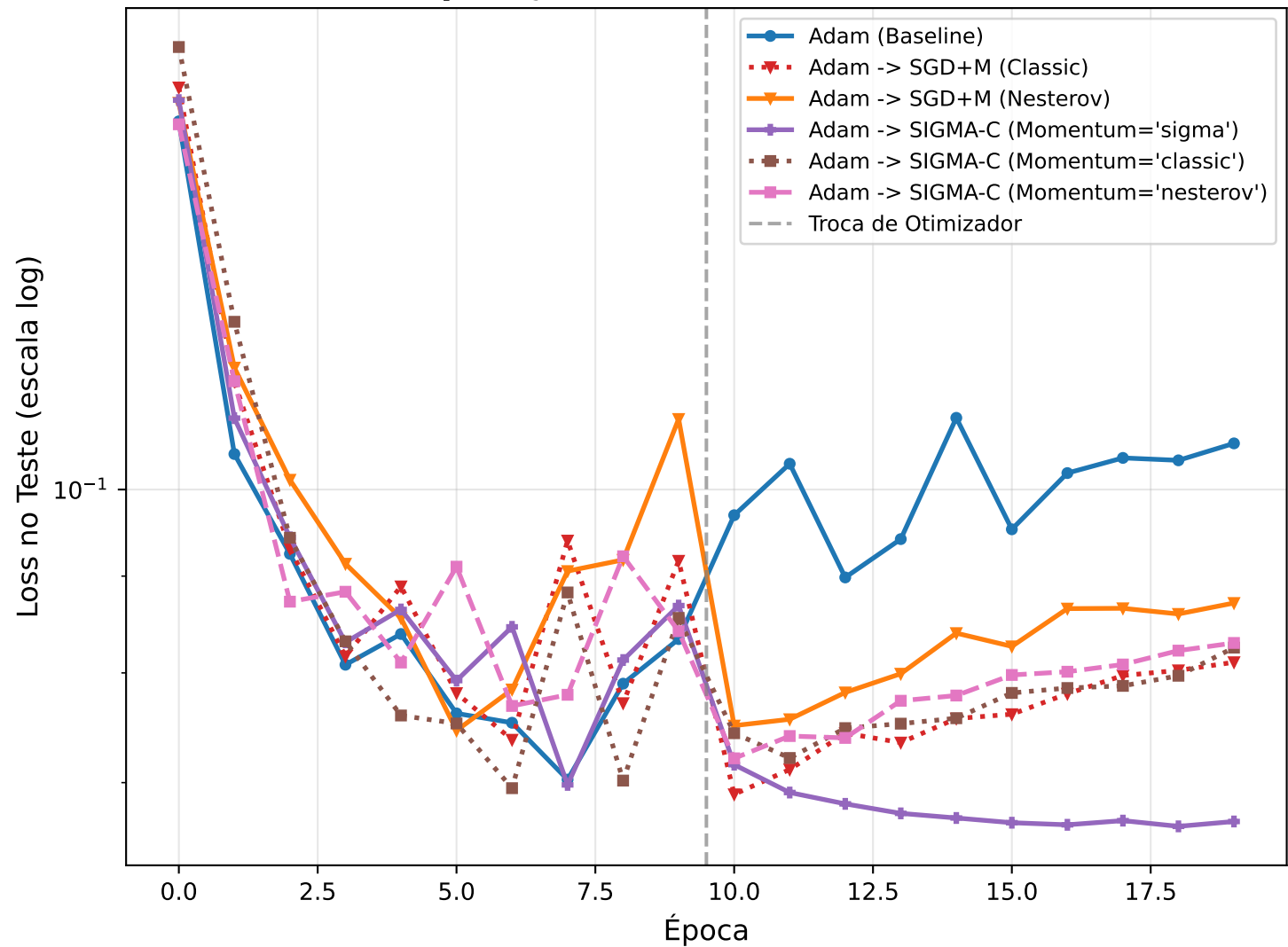
Comparação de Loss (Redes Neurais)
