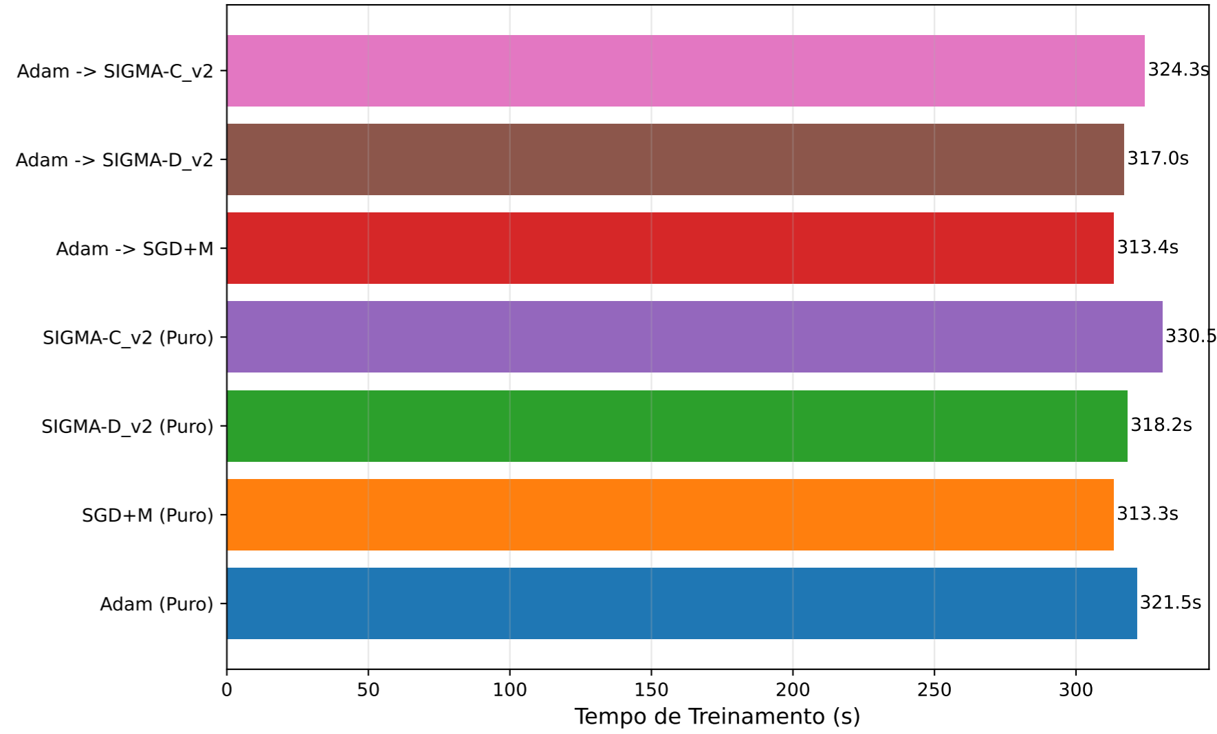
Eficiência Computacional v2 (Regressão Logística)
