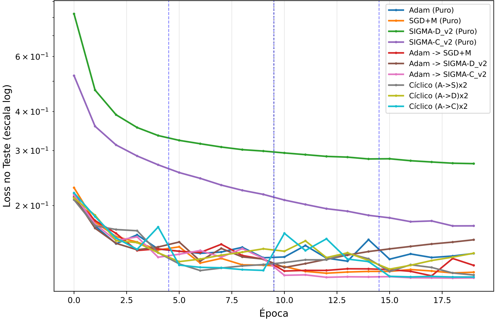
Comparação de Loss v3 (Redes Neurais)
