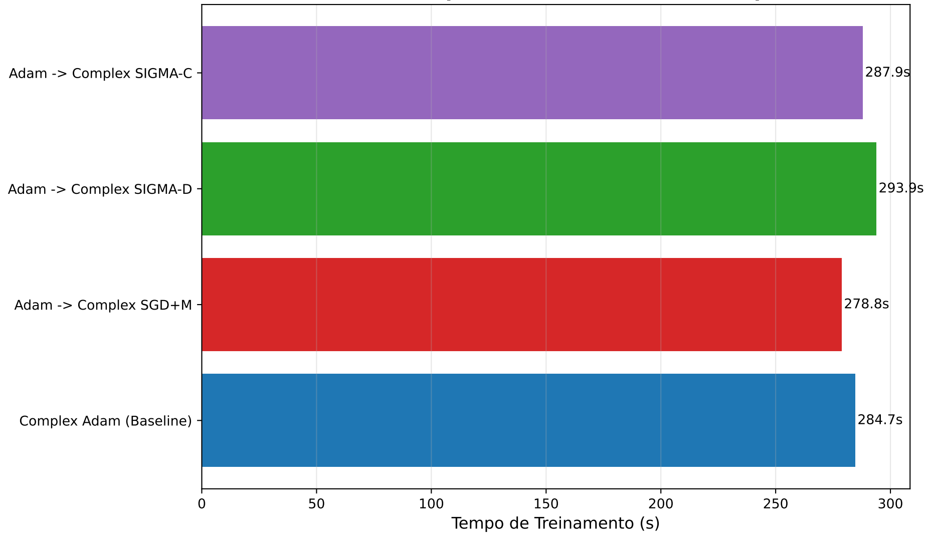
Eficiência Computacional (Rede Neural Complexa)
