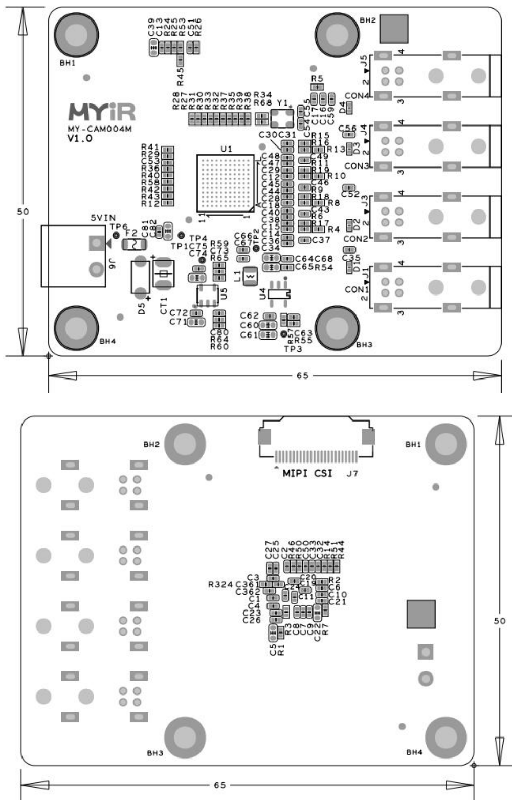
图 5 - 1 MY-CAM004M 尺寸图
