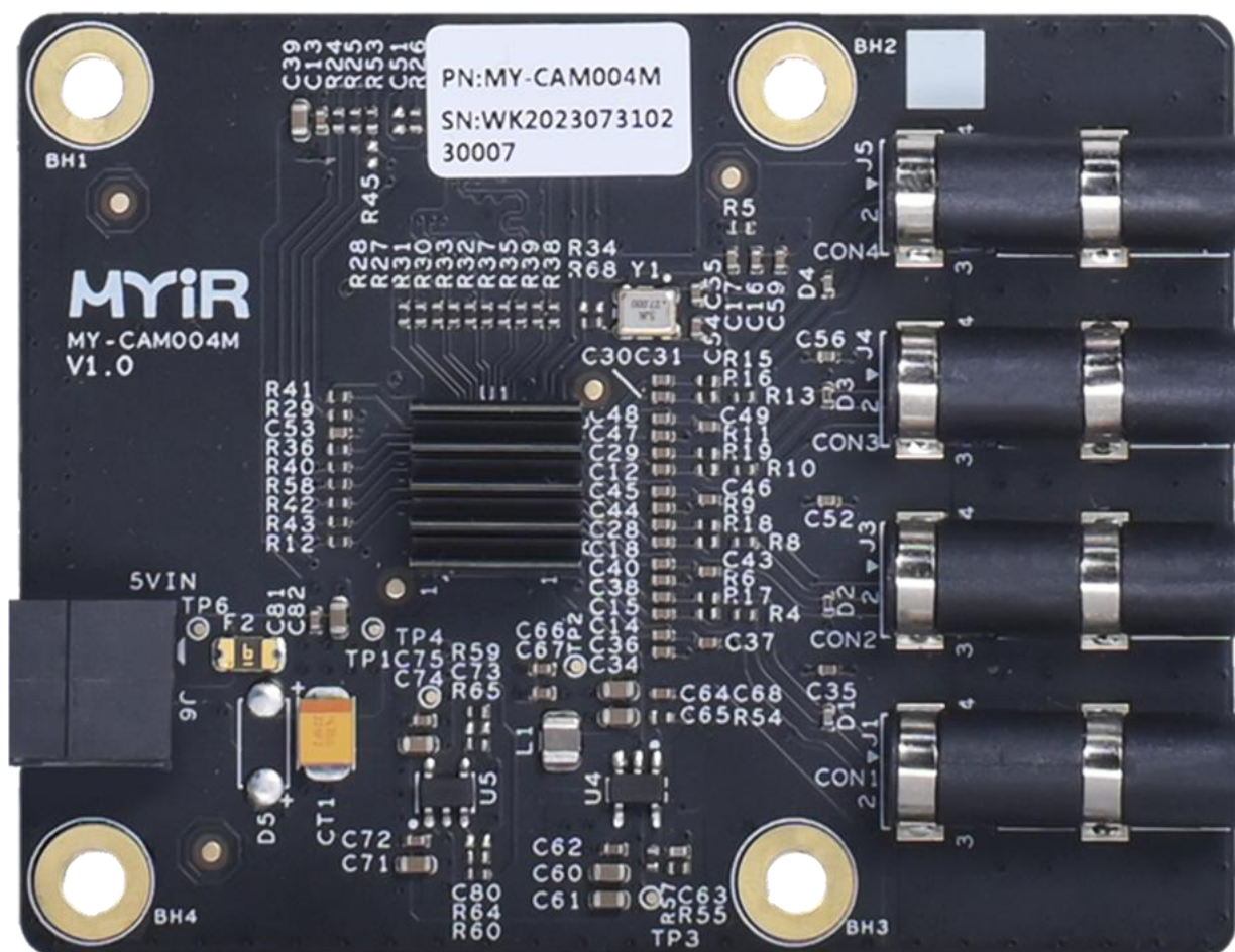
图 1- 1 MY-CAM004M 正面图
