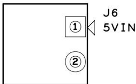
图 3 - 3 J6 引脚顺序图
