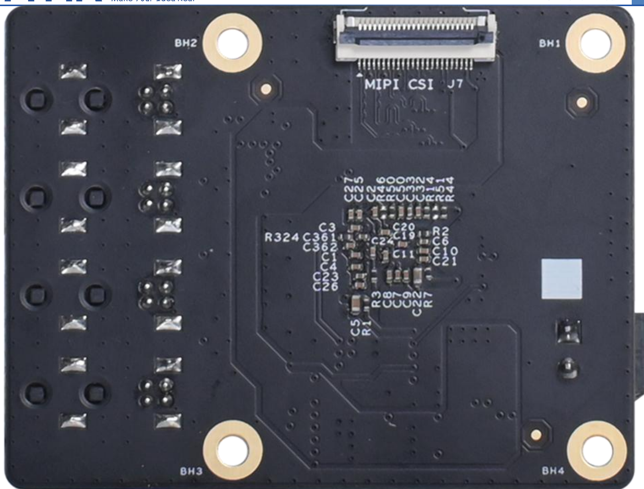
图 1-2 MY-CAM004M 背面图
