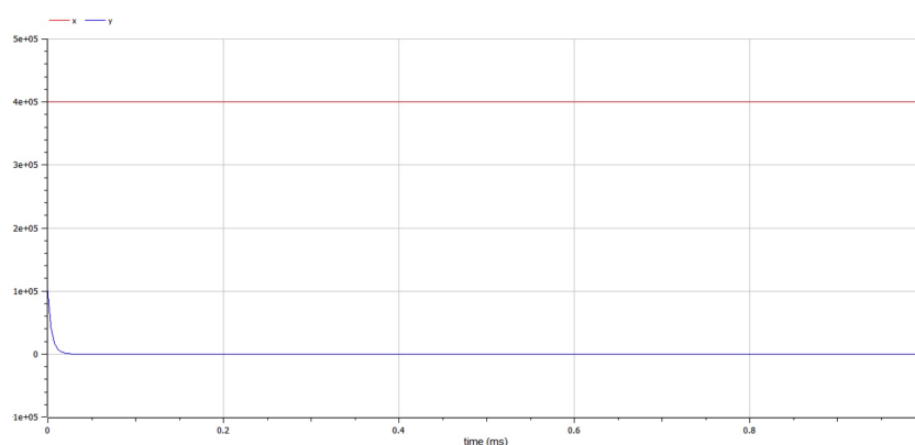
Рис. 4.5: Модель боевых действий с участием регулярных войск и партизанских отрядов
