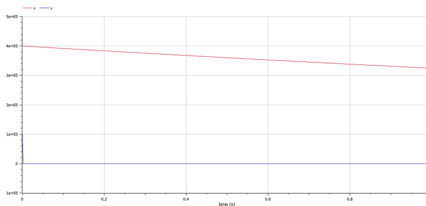
Рис. 4.6: Модель боевых действий с участием регулярных войск и партизанских отрядов
