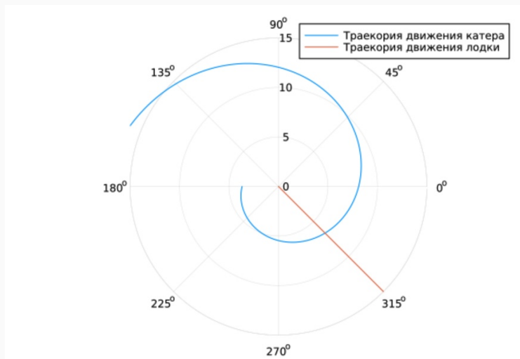
Рис. 4: Траектория движения катера во 2 случае
