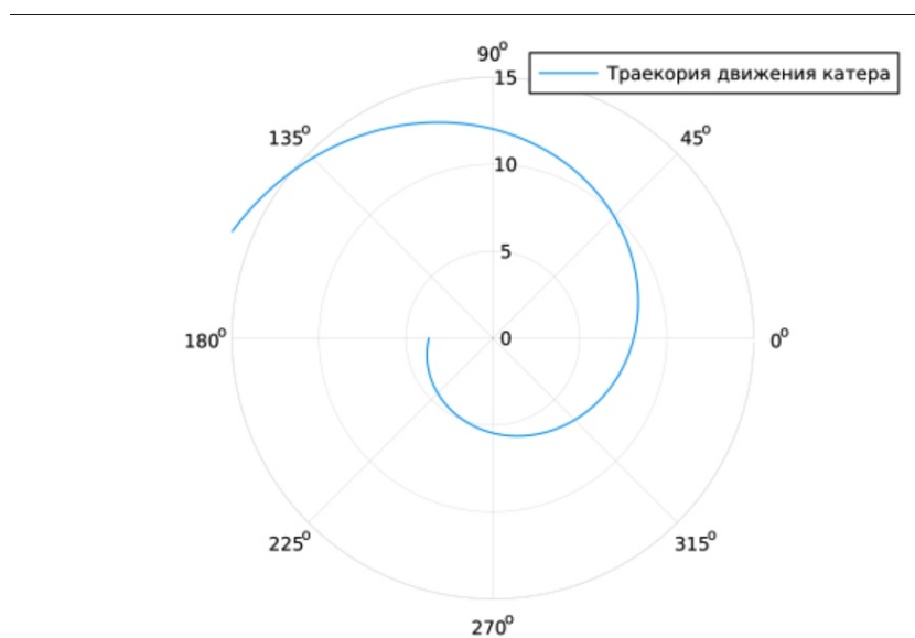
Рис. 4.3: Траектория движения катера во 2 случае
