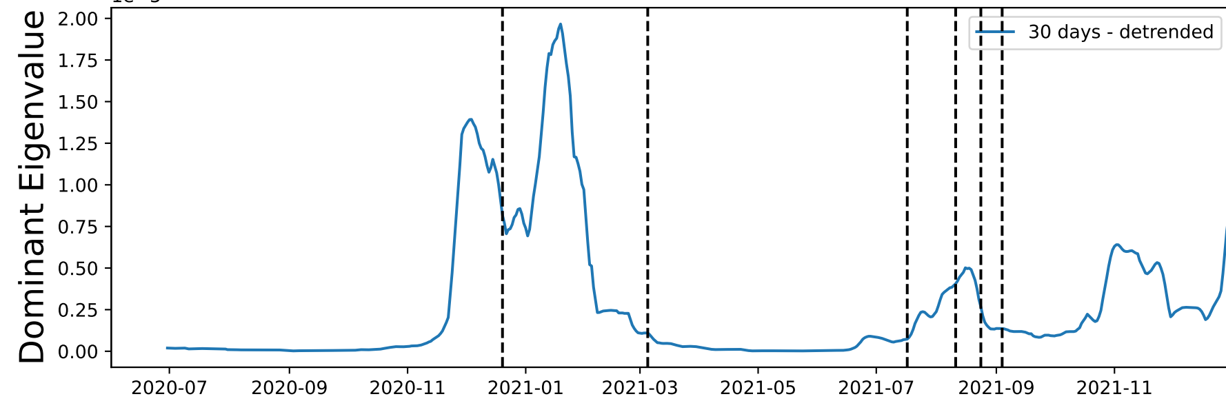
Normalised Eigenvalue
