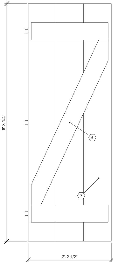
2 DOOR D1 (INSIDE FACE) SCALE: 3/4" = 1'-0"
