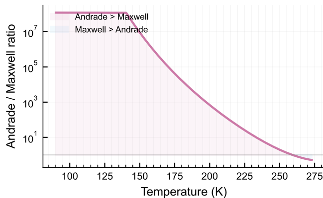
(d) Rheology ratio
