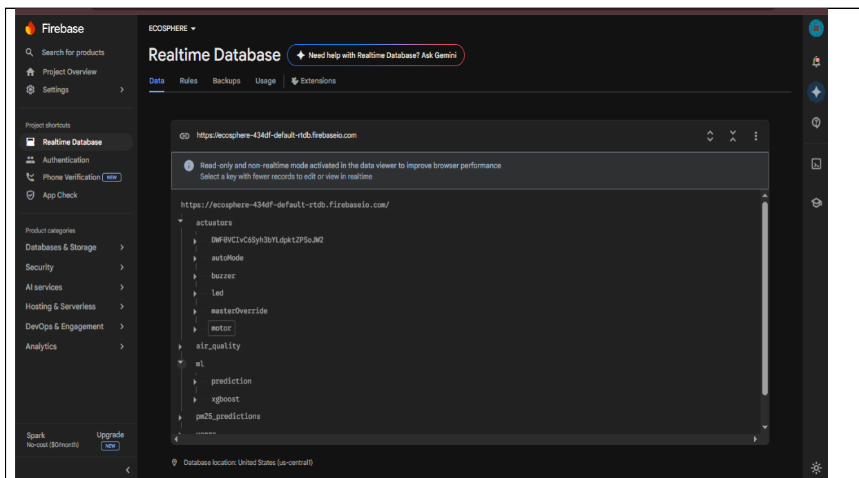
database
