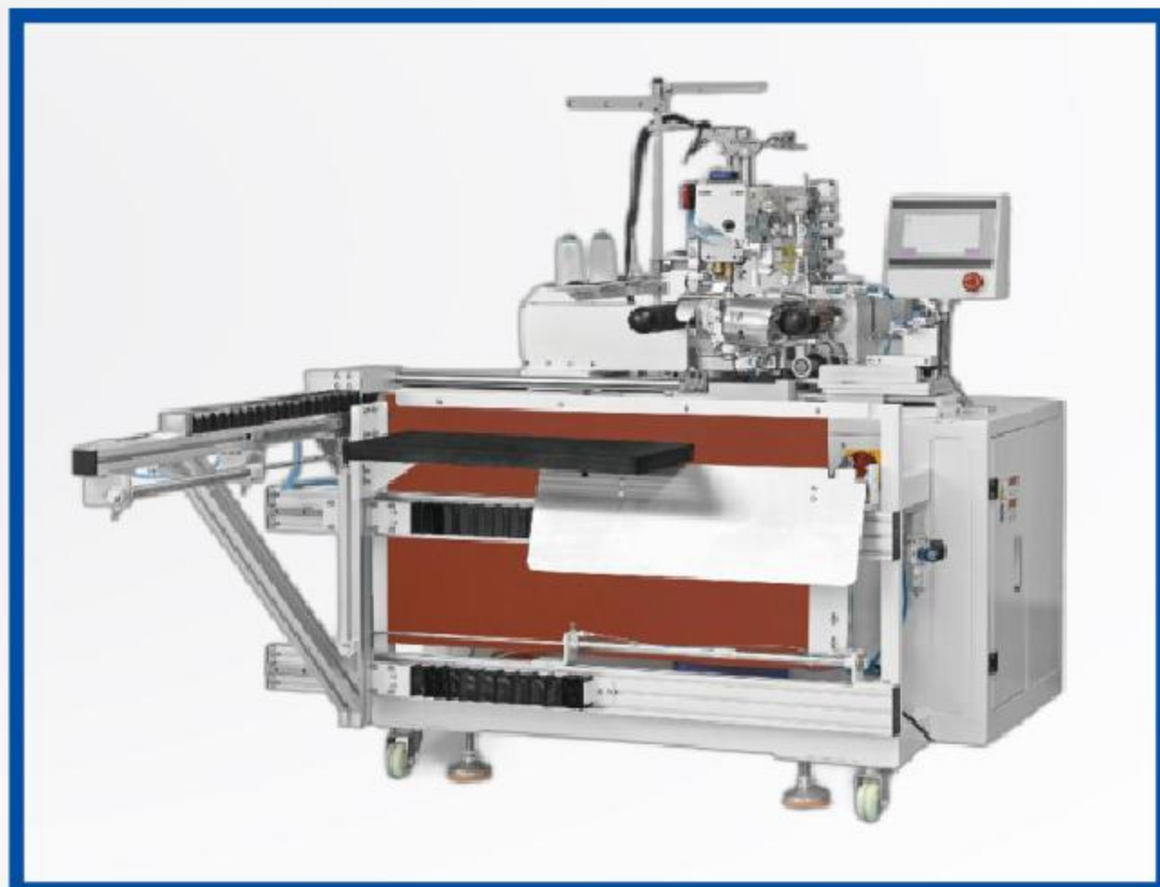
自动童装下摆机器人 AS-300-4 Automatic CoverStitch Bottom Hemmer
