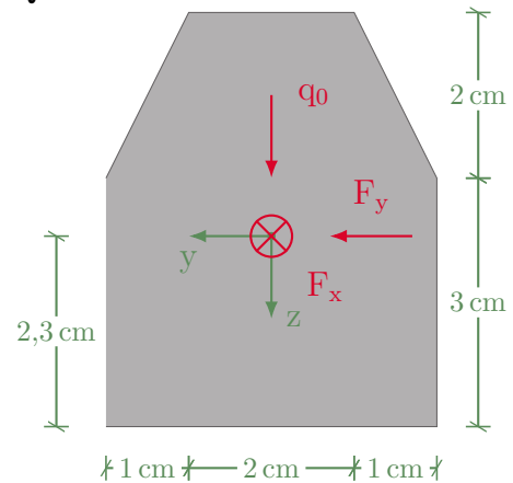
Querschnitt:
