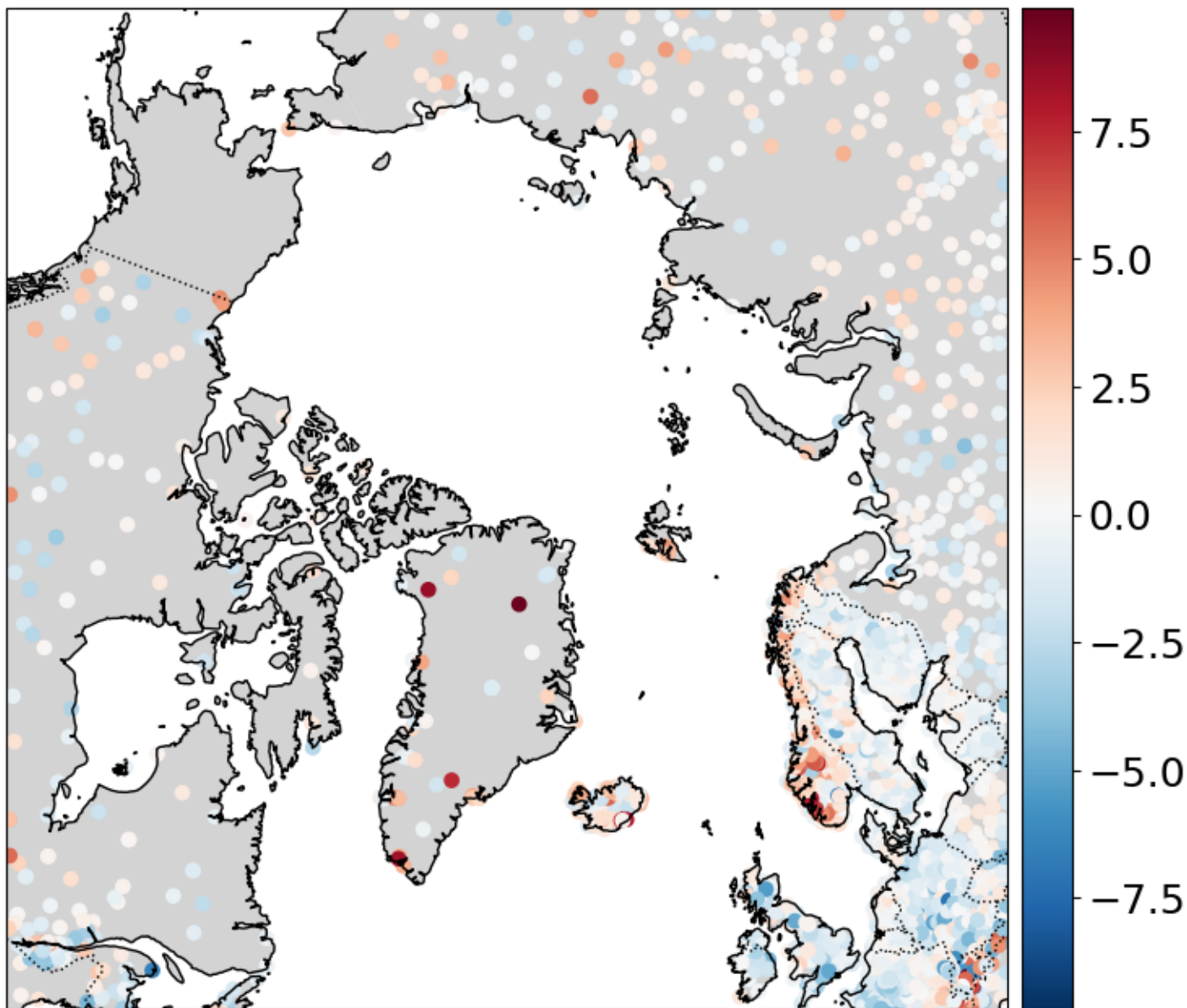
T2M OmF
