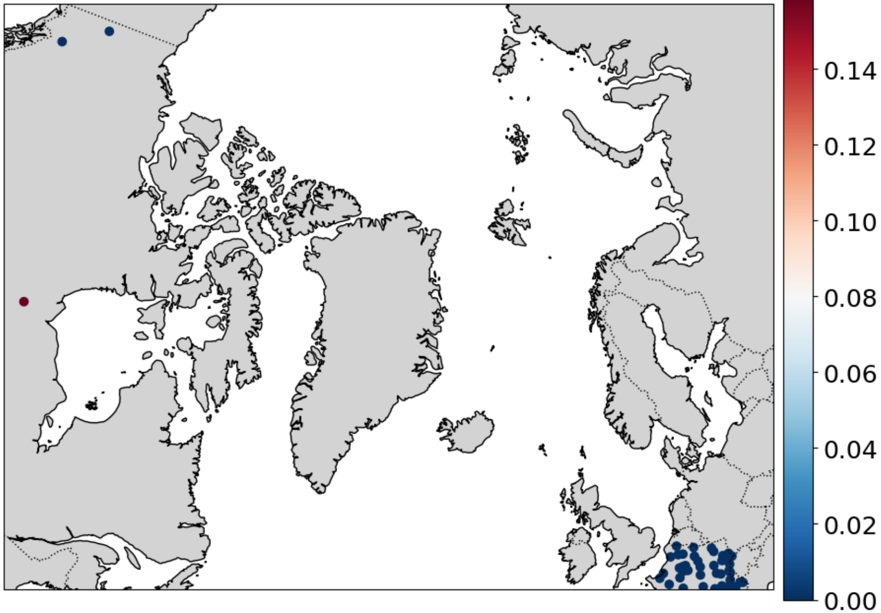
SD OmF
