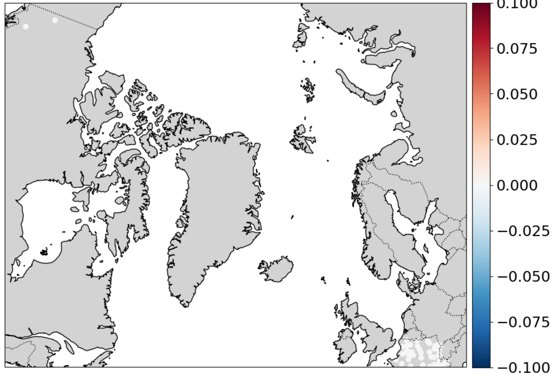
SD OmF
