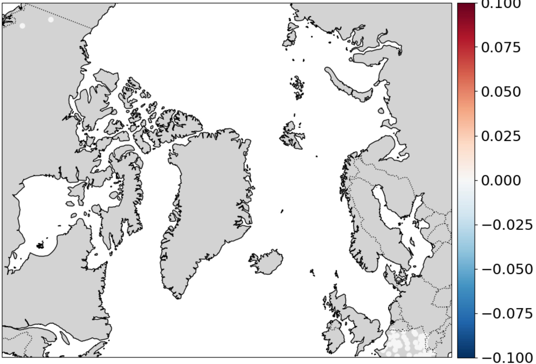
SD OmF
