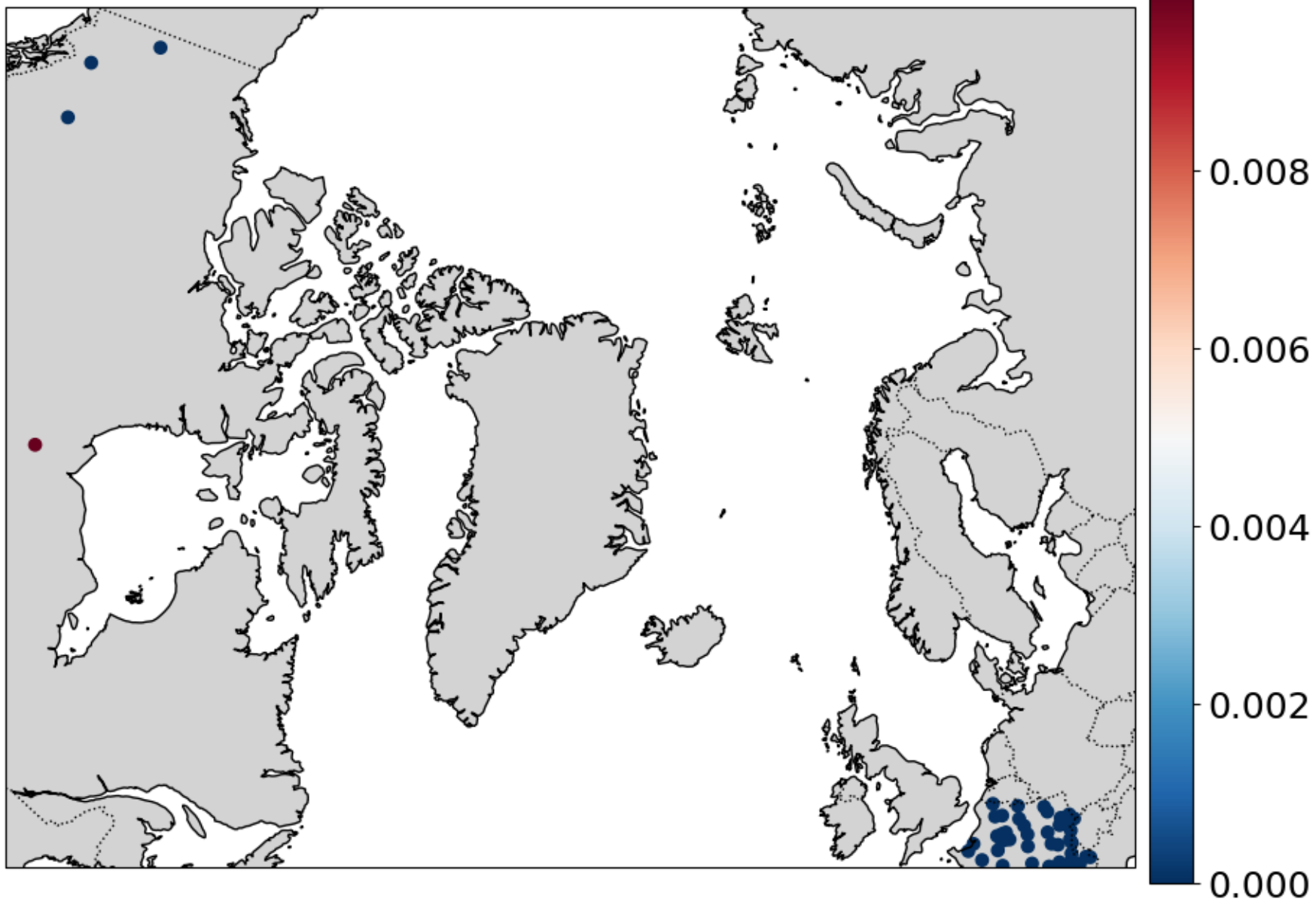
SD OmF
