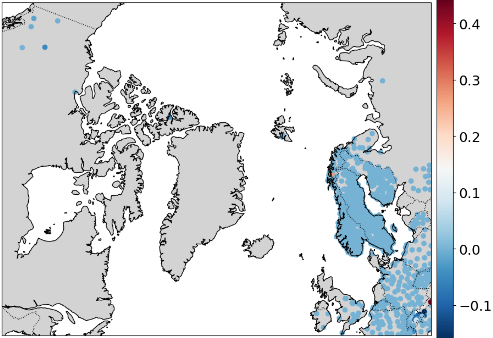
SD OmF
