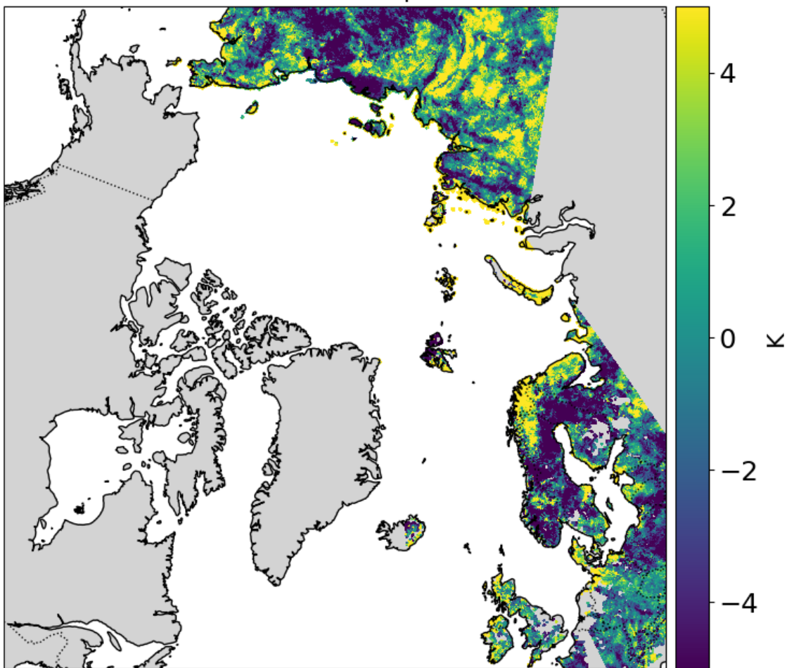
OmF 18GHz V-pol
