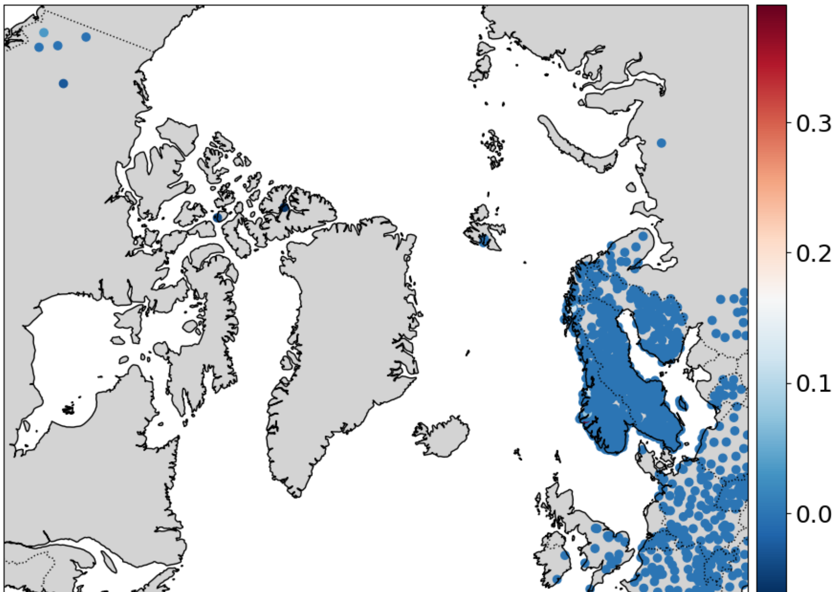
SD OmF
