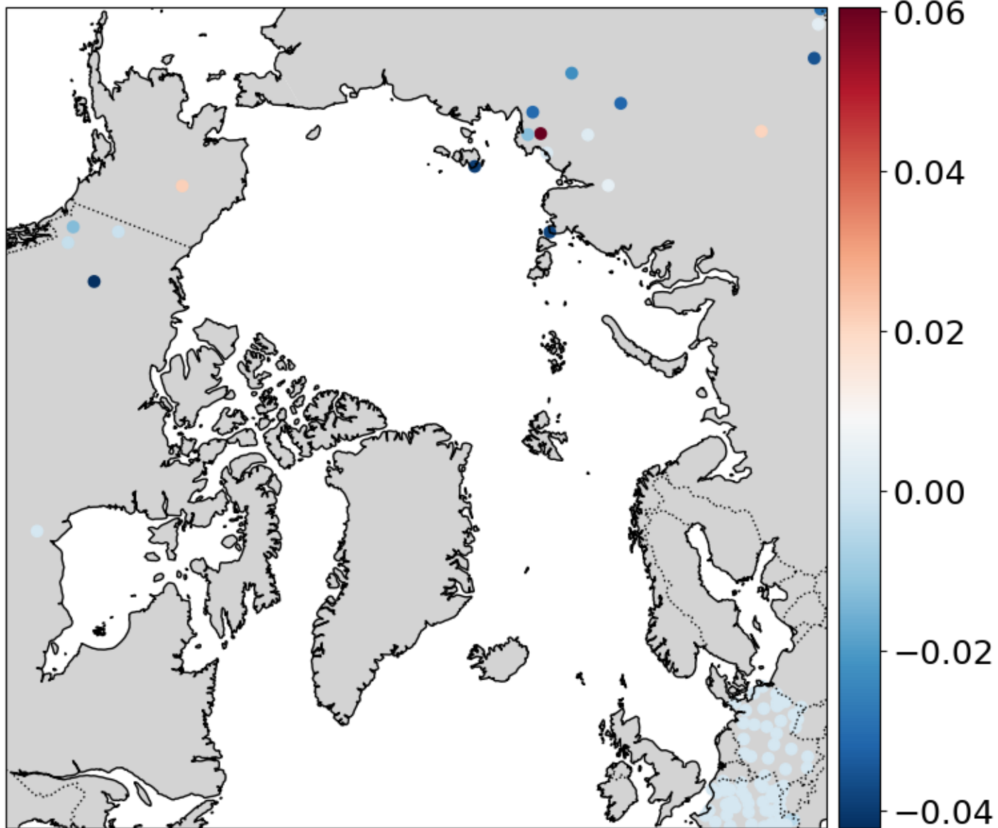
SD OmF
