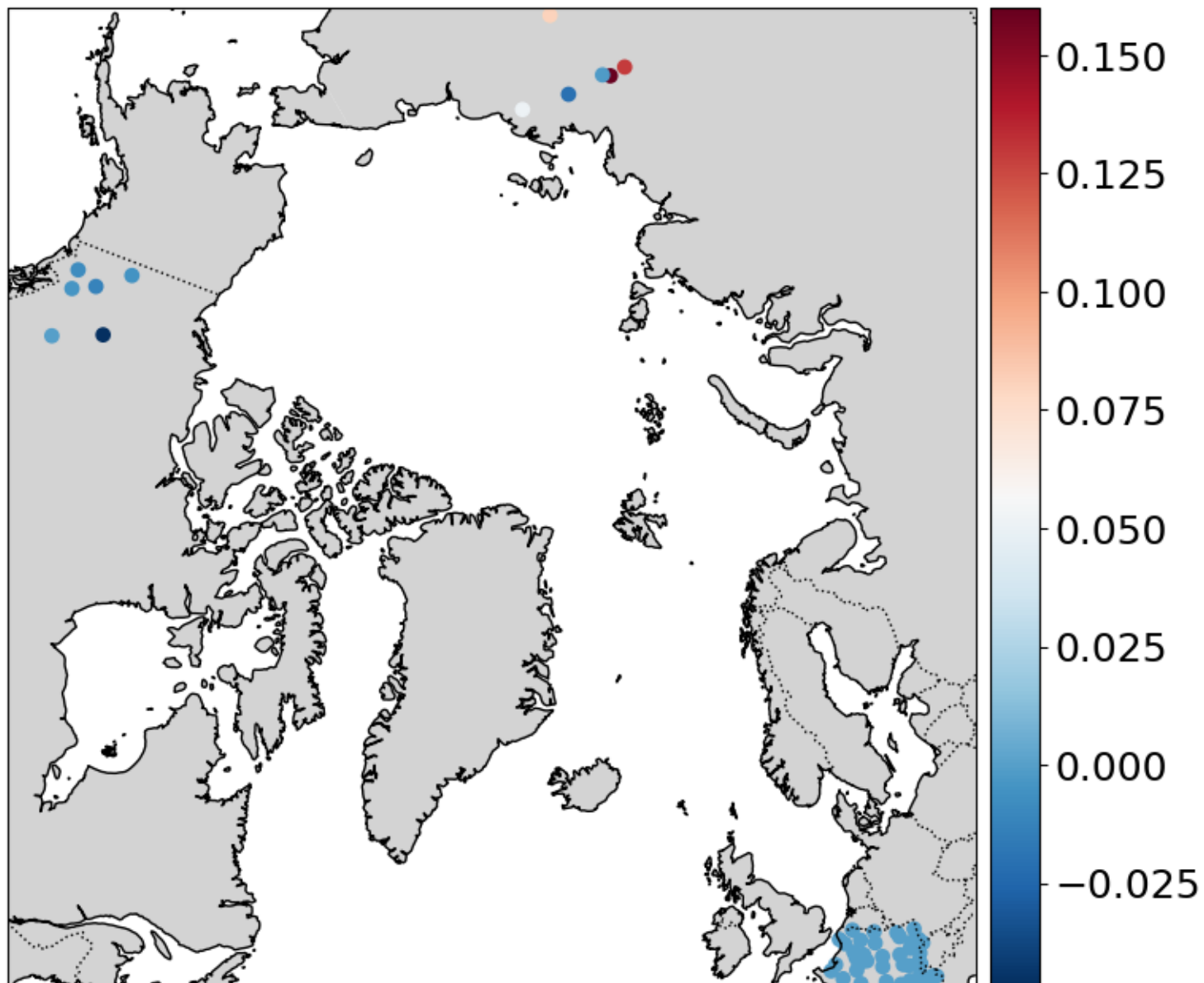
SD OmF
