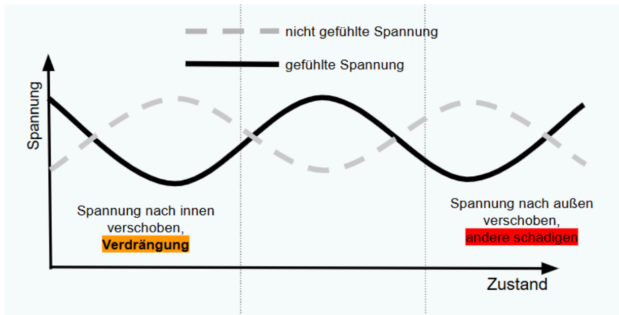
Abbildung 11: Verdrängungsspannung
