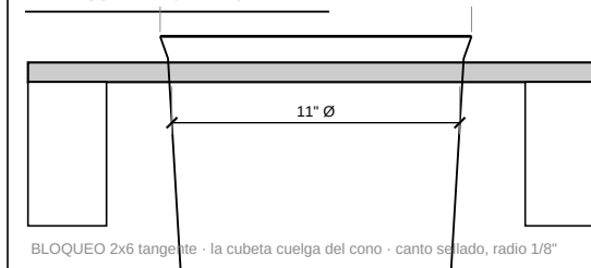
4 DETALLE DEL HUECO ESCALA: 1 1/2" = 1'-0"
