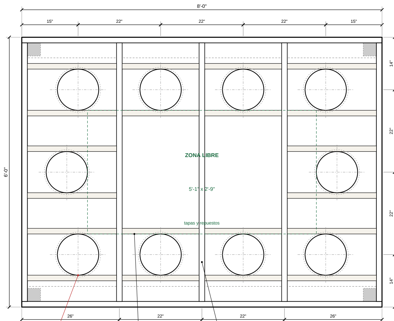
3 PLANTA DE LA PLATAFORMA ESCALA: 3/4" = 1'-0"
