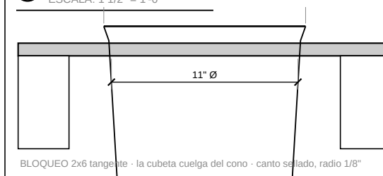
4 DETALLE DEL HUECO ESCALA: 1 1/2" = 1'-0"
