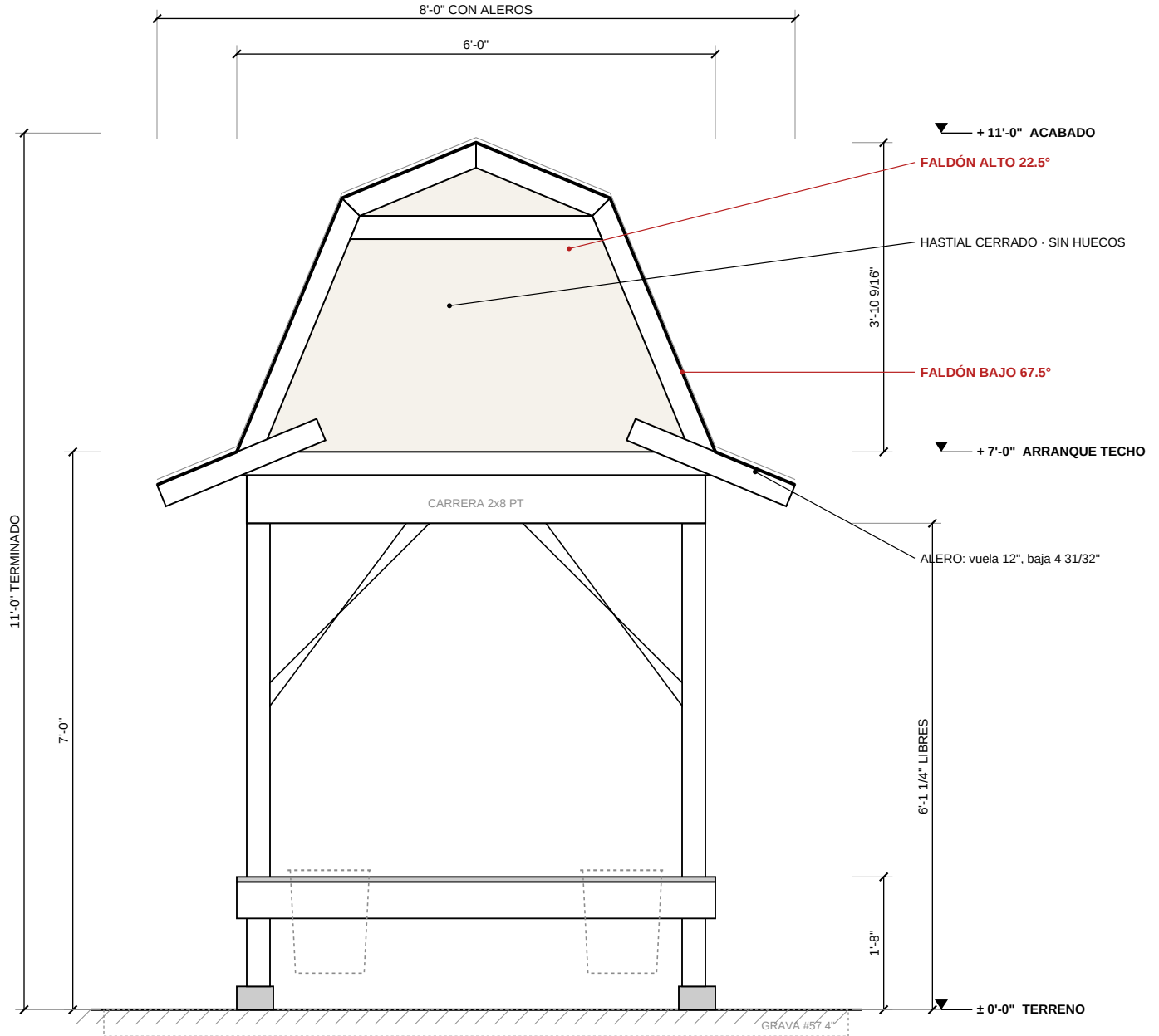
① ALZADO FRONTAL ESCALA: 1/2" = 1'-0"
