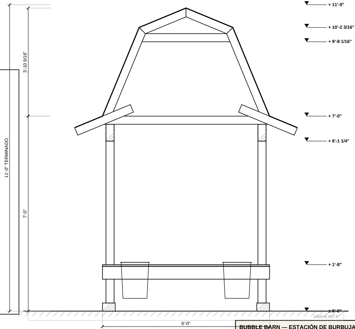
5 SECCIÓN TRANSVERSAL ESCALA: 1/2" = 1'-0"
