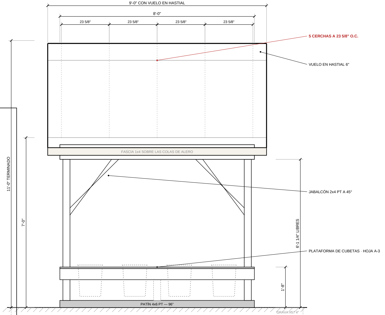
② ALZADO LATERAL ESCALA: 1/2" = 1'-0"
