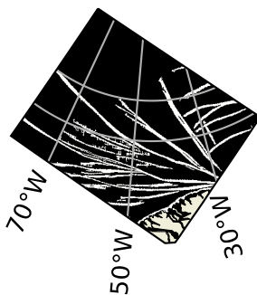
e) SEDNA Lead mask
