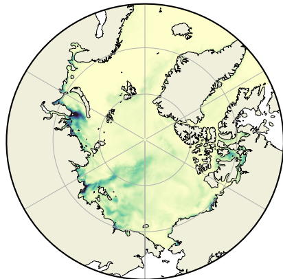
c) SEDNA: variance MLD density
