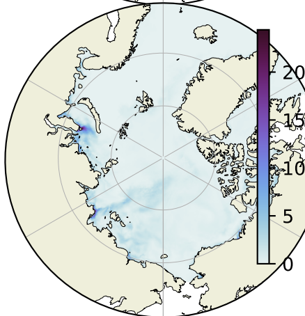
c) SEDNA: variance MLD density
