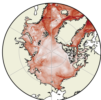
g) SEDNA: kinetic energy at 5m depth
