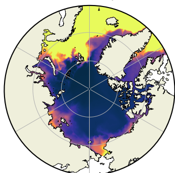
e) SEDNA: salinity at 5m depth
