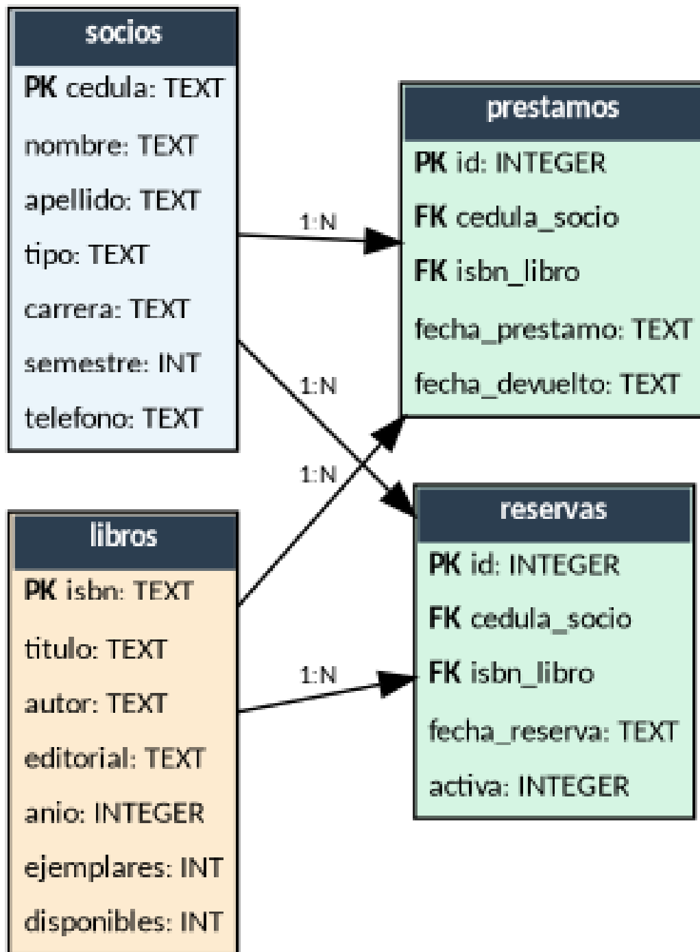
*Diagrama 2: Modelo entidad-relación de la base de datos mostrando las 4 tablas (socios, libros, prestamos, reservas), sus atributos, tipos de datos, claves primarias (PK) y foráneas (FK), y las relaciones 1:N entre ellas.*
