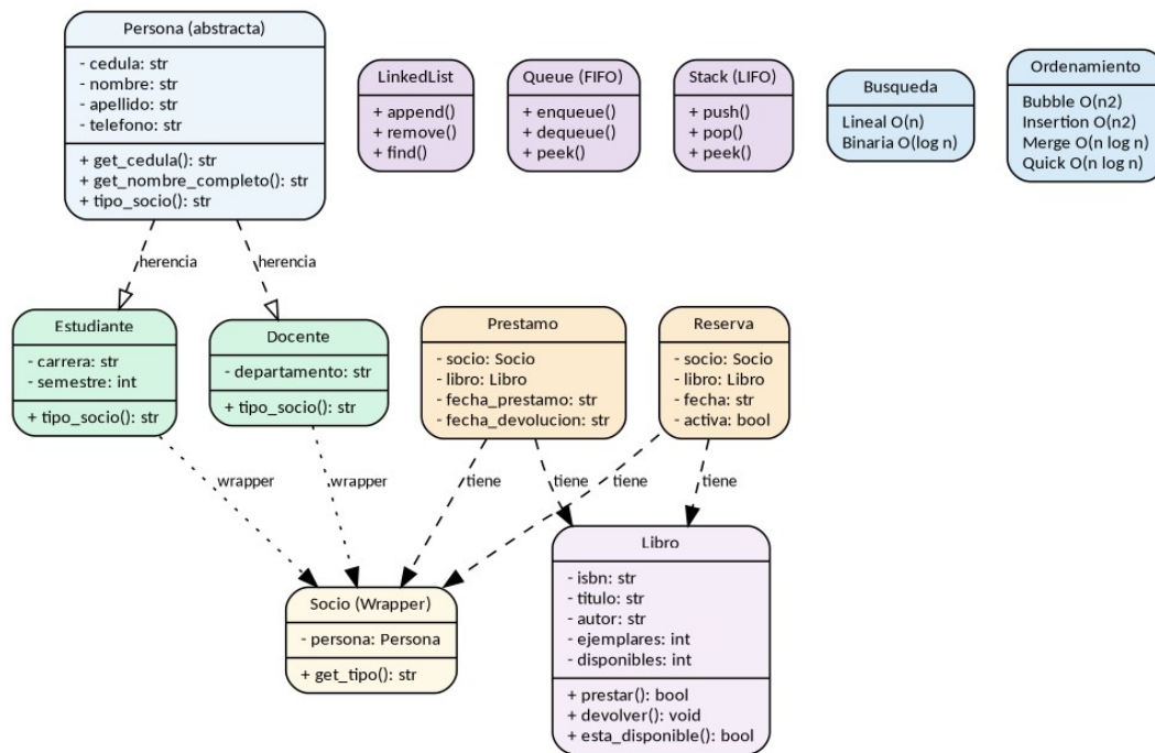
*Diagrama 1: Diagrama de clases del sistema mostrando jerarquía de herencia (Persona → Estudiante/Docente), wrapper polimórfico (Socio), modelos de dominio (Libro, Prestamo, Reserva), estructuras de datos (LinkedList, Queue, Stack) y algoritmos de búsqueda y ordenamiento.*
