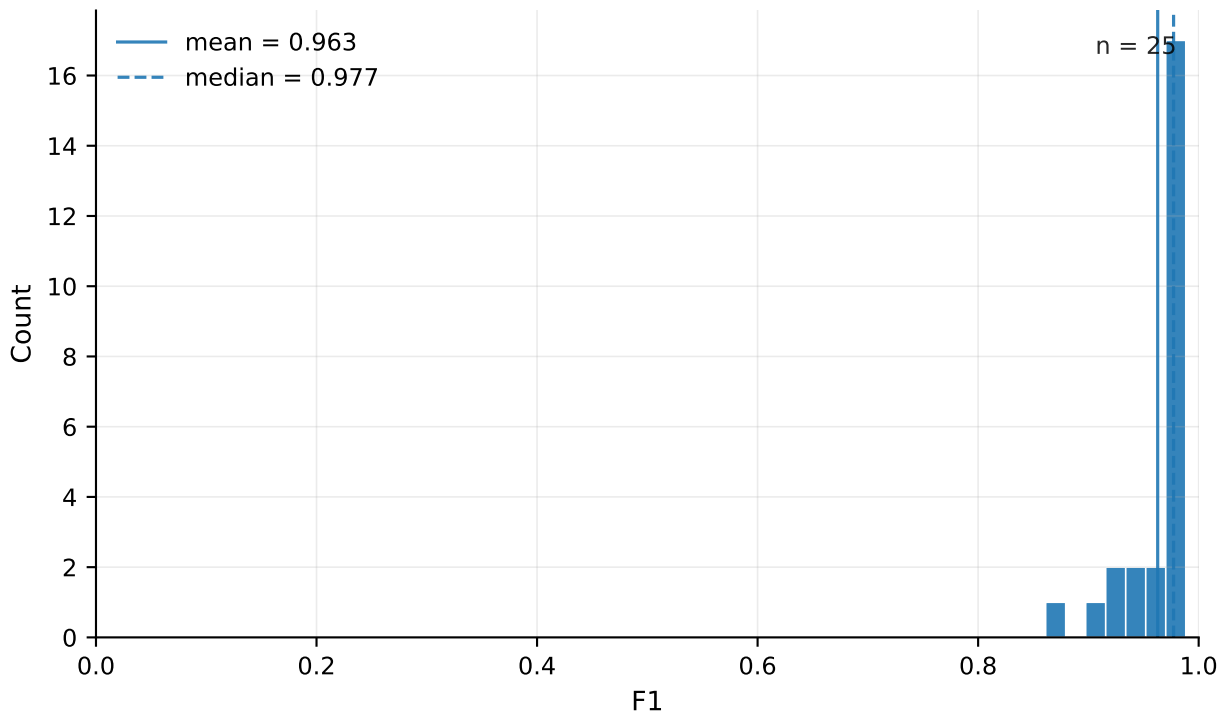
F1 distribution
